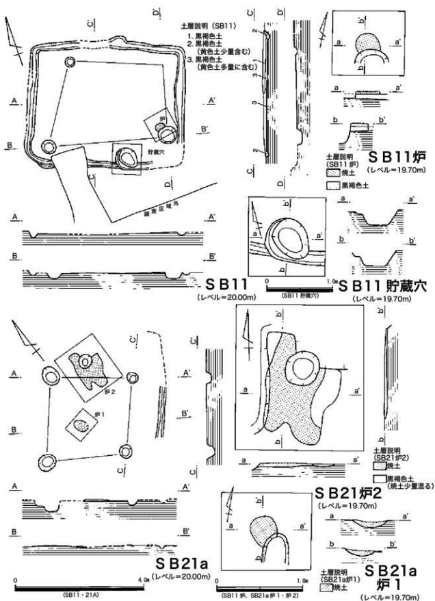
第118図 第85-1・90・94次 SB11・21a 実測図
