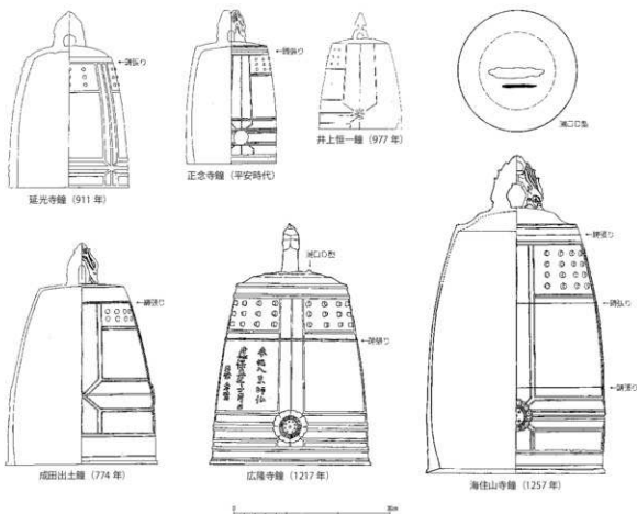
図 29 小型鐘と簡易な装束樺、瀬口 D 型資料 (杉山編 1993、五十川 2009 より)
