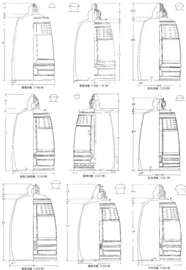
図 25 - 2 本鐘と年代に近い有銘鐘実測図 2 (杉山編 1993 年より抽出、縮尺不同)
