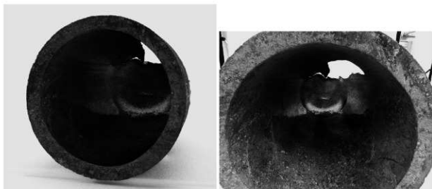
図 22 梵鐘内面に残る埋没痕跡と水没痕跡
