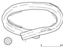
図 14 鉄製吊金具写真・実測図 (1/3)
