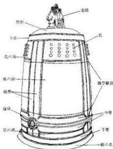
図6 梵鐘各部名称（坪井 1993）
