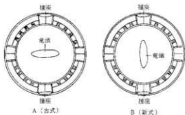
図 12 龍頭の方向と撞座の位置関係 (坪井 1993)
