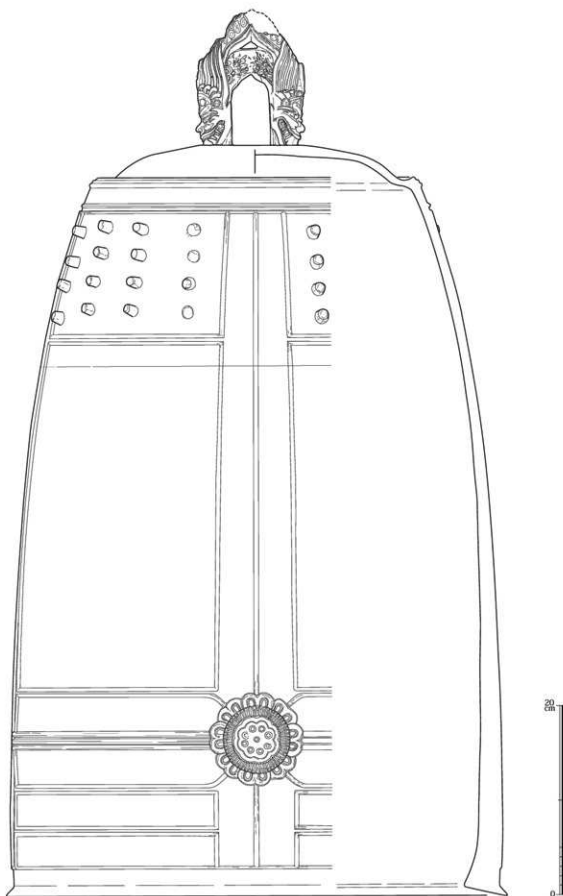
図8 平治二年銘梵鐘実測図 (1/4)
