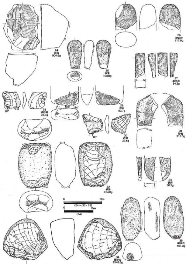
第47図 第60次 石製品実測図2
