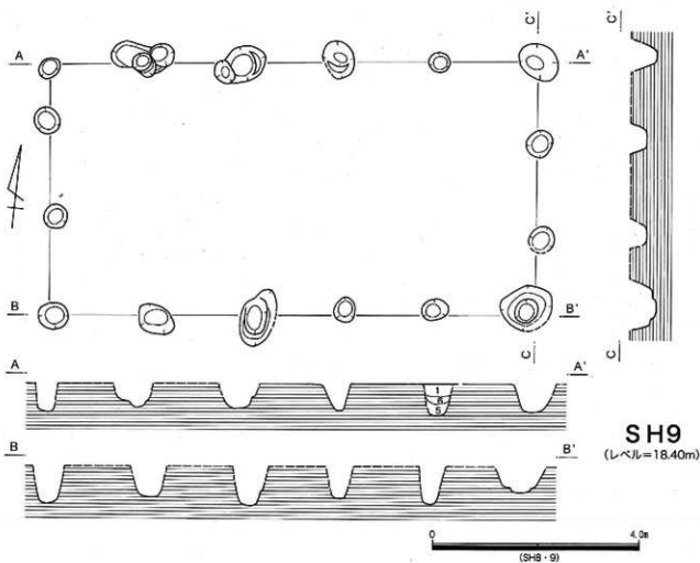
第106図 第63・75-1次 SH8・9実測図
