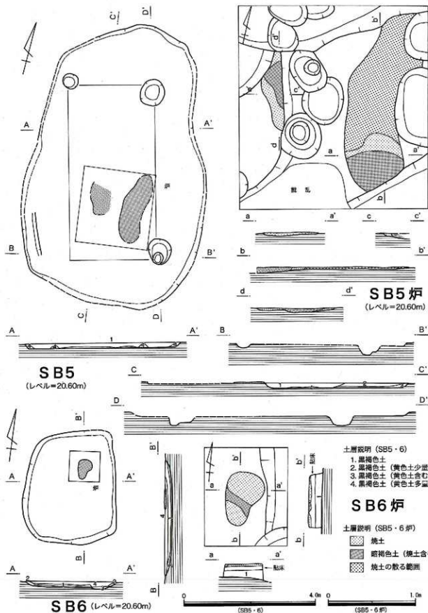
第51図 第61・72・74次 SB5・6実測図
