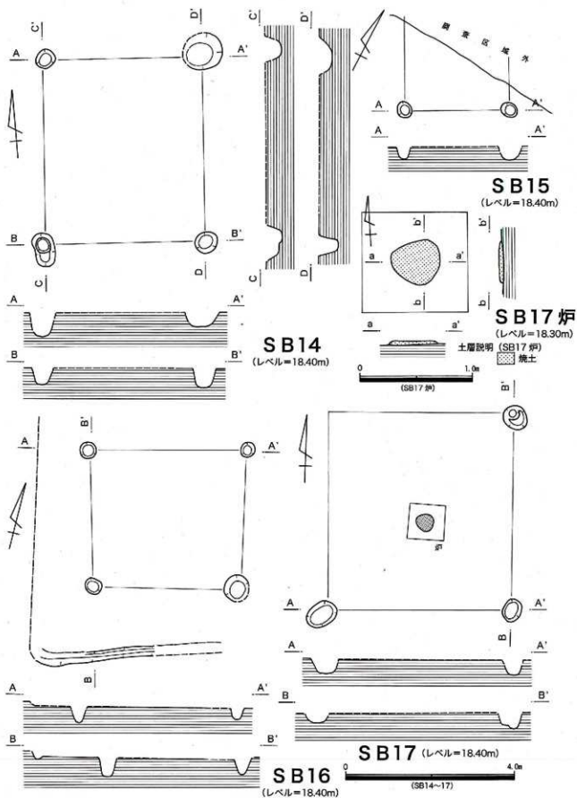
第104図 第63・75-1次 SB14~17実測図
