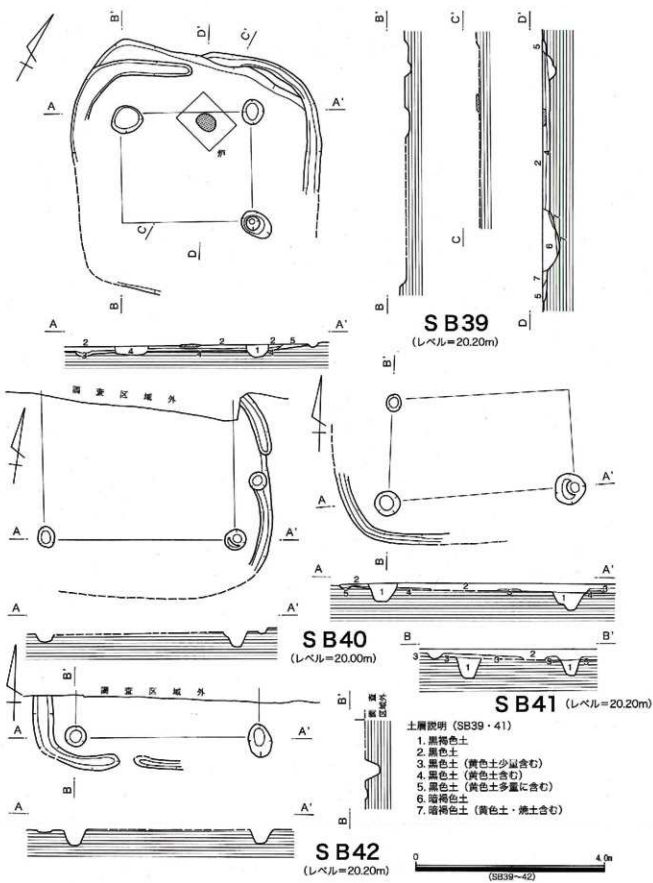
第33図 第60次 SB39～42実測図
