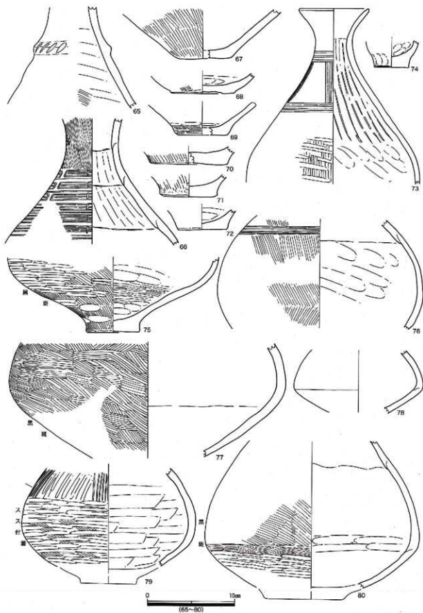
第92図 第62次 土器実測図3
