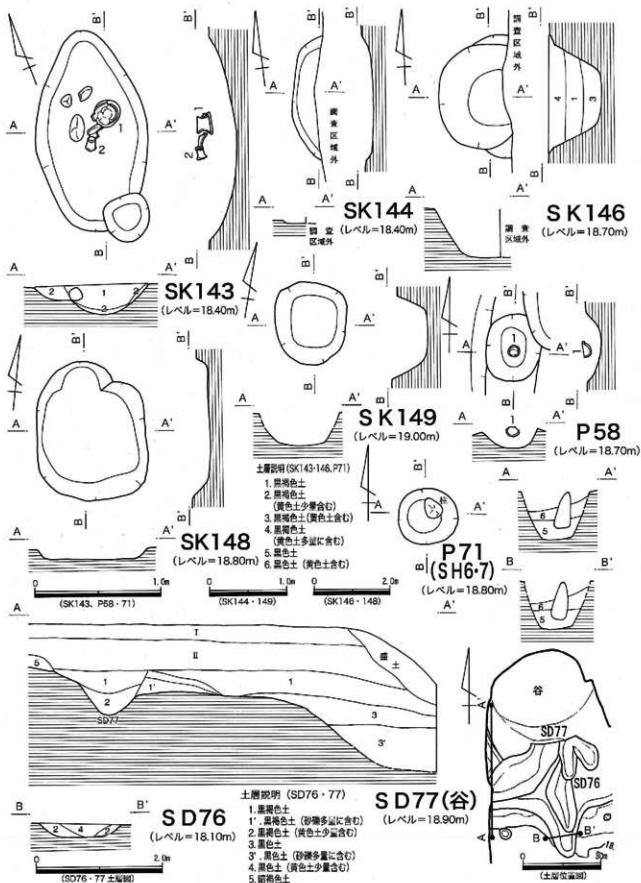
第89図 第62次 SK143・144・146・148・149、P58・71実測図、D76・77土層図
