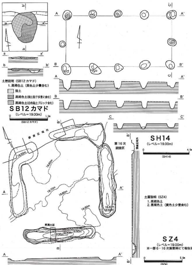
第6図 第57次 SB12カマド・SH14・SZ4実測図
