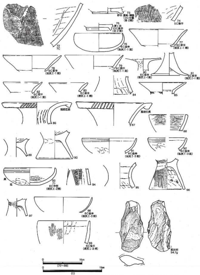
第23図 第58・77次 土器実測図4、石製品実測図
