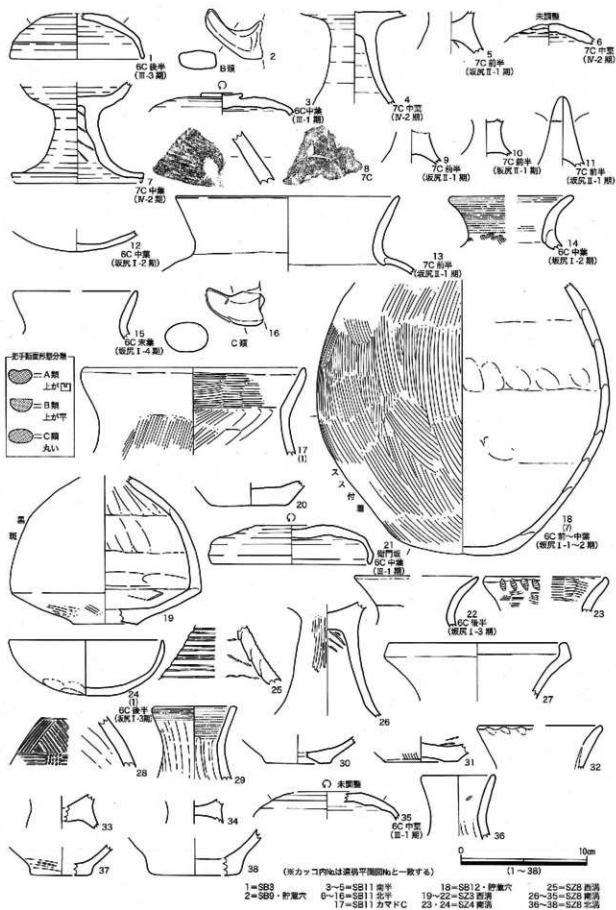
第10図 第57次 土器実測図1
