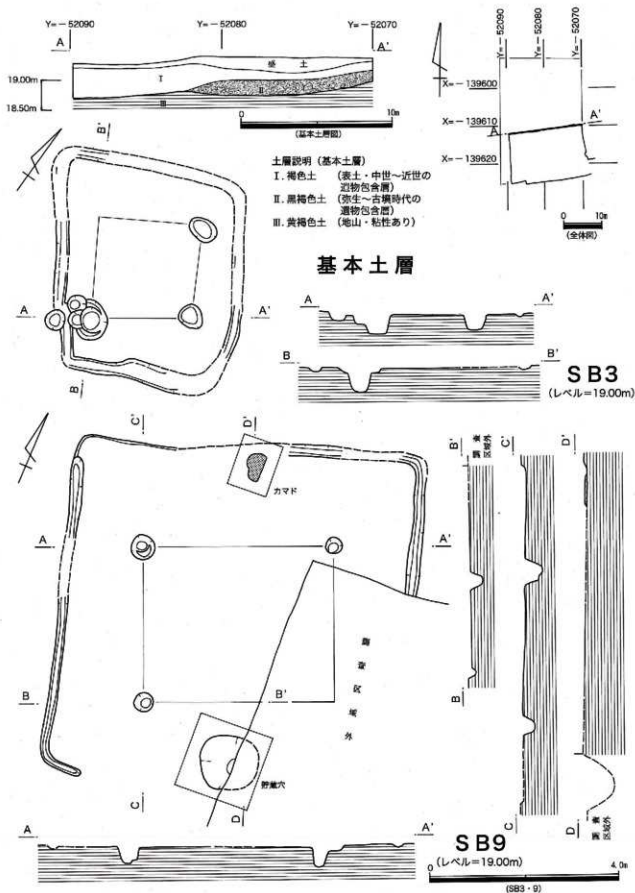
第3図 第57次 基本土層図、SB3・9実測図
