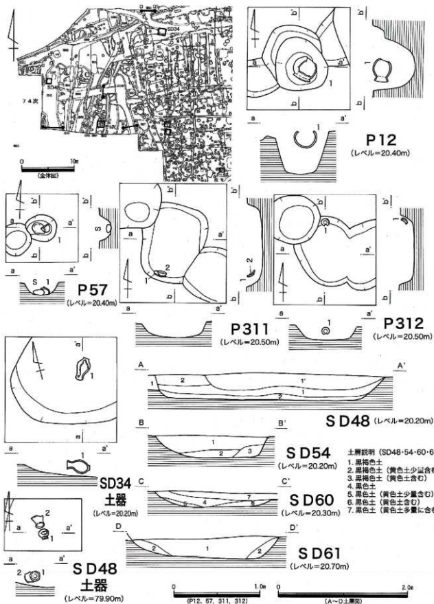
第62図 第61・72・74次 P12・57・311・312、SD34・48土器出土状況図、SD54・60・61土層図
