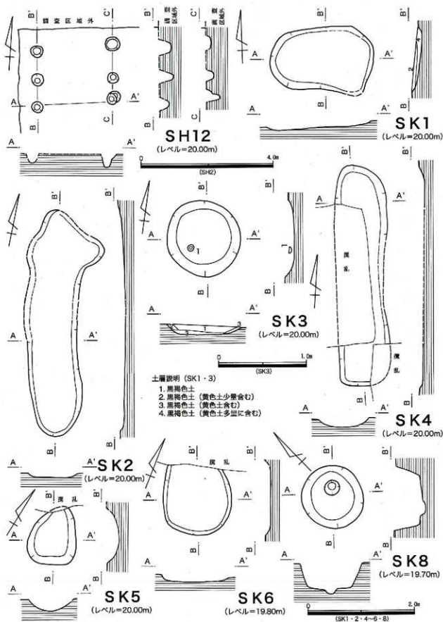
第28図 第59次 SH12、SK1~6・8実測図
