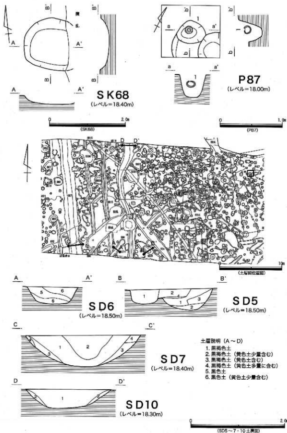
第110図 第63・75-1次 SK68、P87実測図、SD5~7・10土層図
