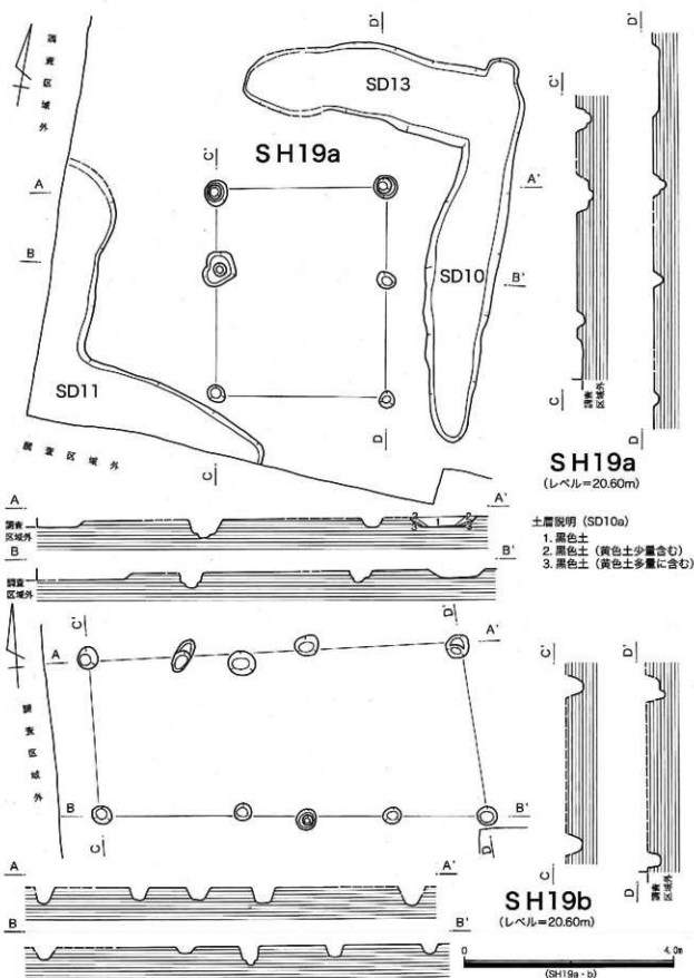
第55図 第61・72・74次 SH19a・SH19a・b実測図
