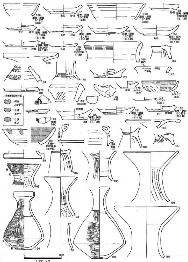
第96図 第62次 土器実測図7
