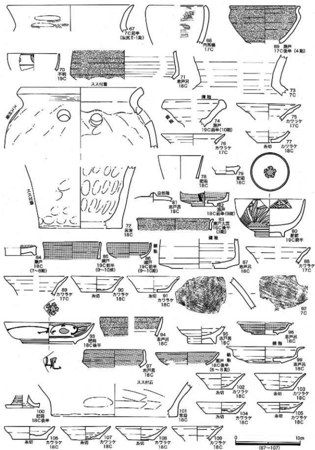
第12図 第57次 土器実測図3
