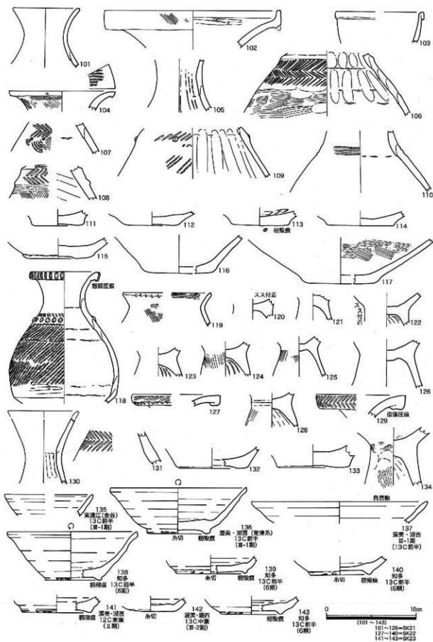
第66図 第61・72・74次 土器実測図4
