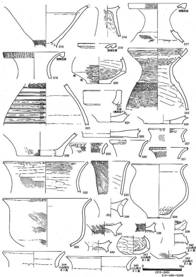
第72図 第61・72・74次 土器実測図10
