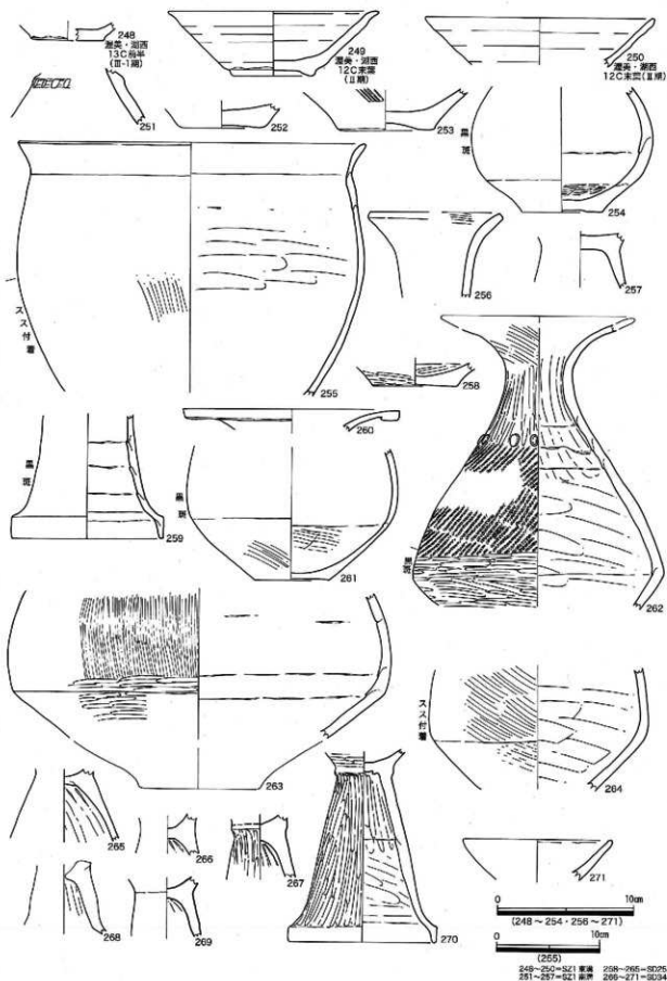
第70図 第61・72・74次 土器実測図8
