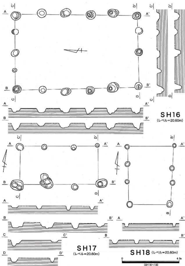
第54図 第61・72・74次 SH16～18実測図
