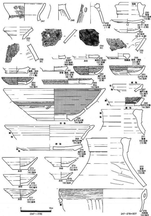
第119図 第63・75-1次 土器実測図9
