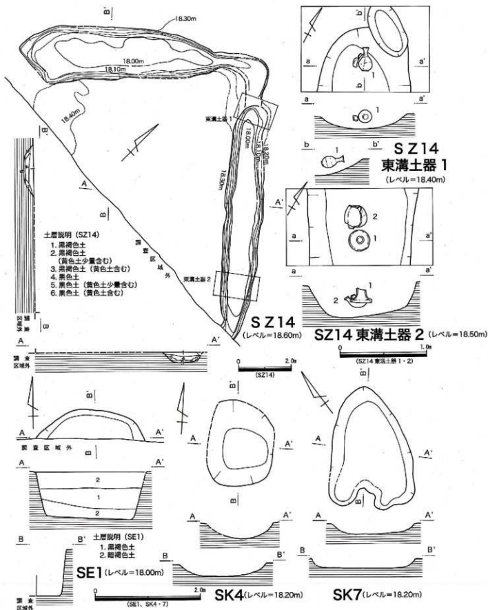
第107図 第63・75-1次 SZ14、SE1、SK4・7実測図
