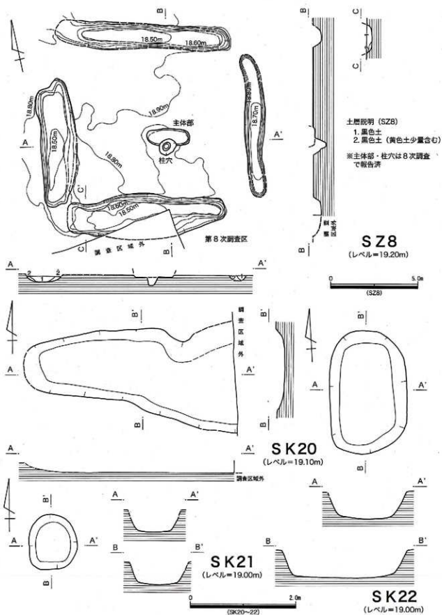
第8図 第57次 SZ8、SK20～22実測図
