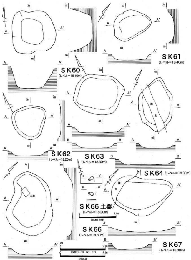
第109図 第63・75-1次 SK60～64・66・67実測図
