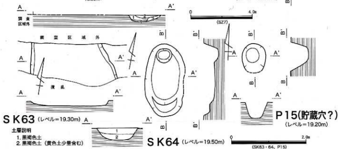
第18図 第58・77次 SZ7、SK63・64、P15実測図
