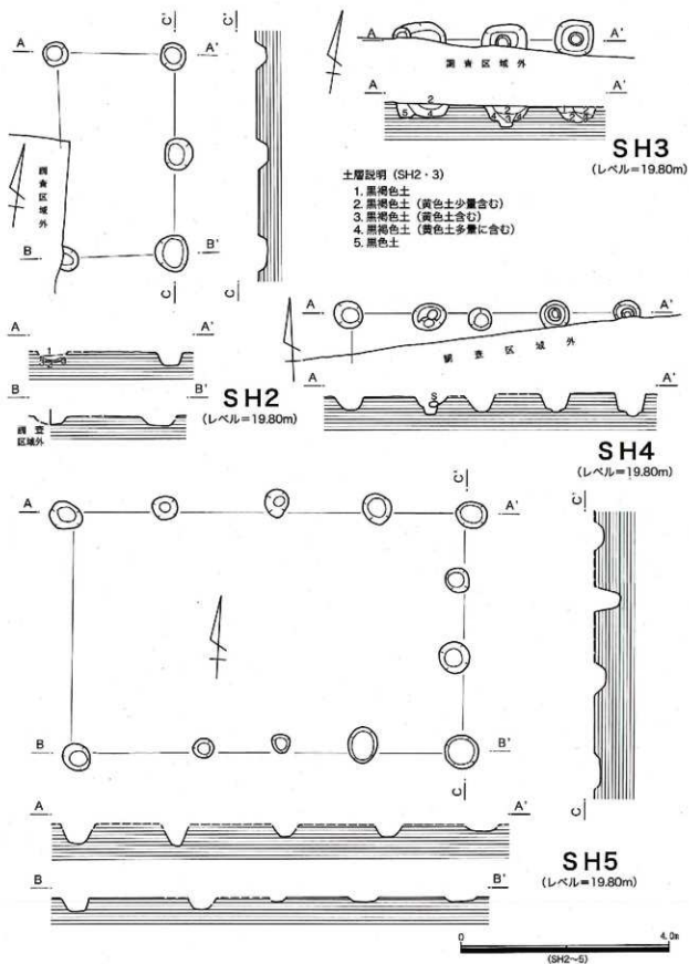
第26図 第59次 SH2~5実測図
