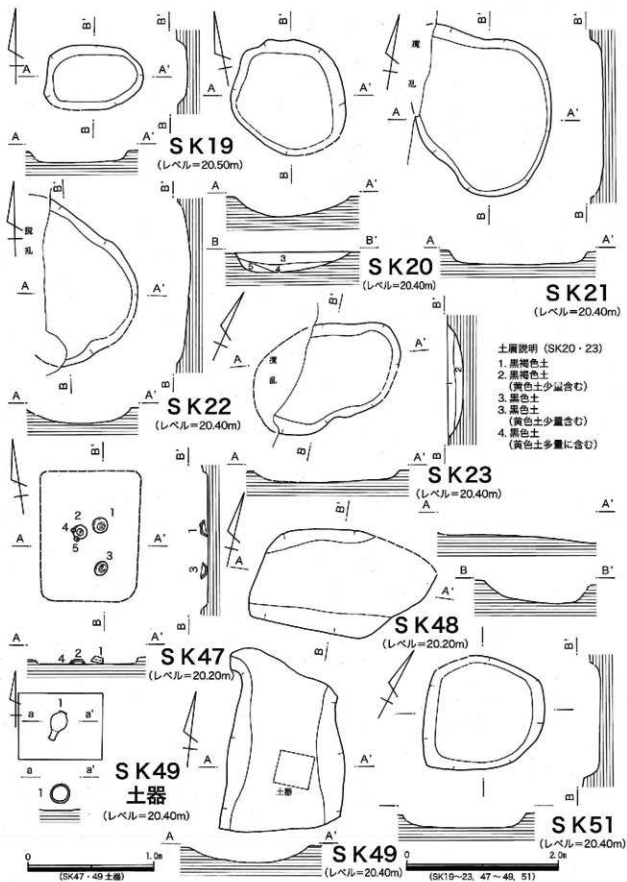
第61図 第61・72・74次 SK19~23・47~49・51実測図
