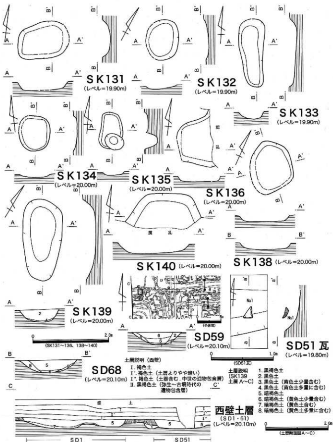
第35図 第60次 SK131~136・138~140、SD51瓦出土状況図、SD59・68・西壁土層図
