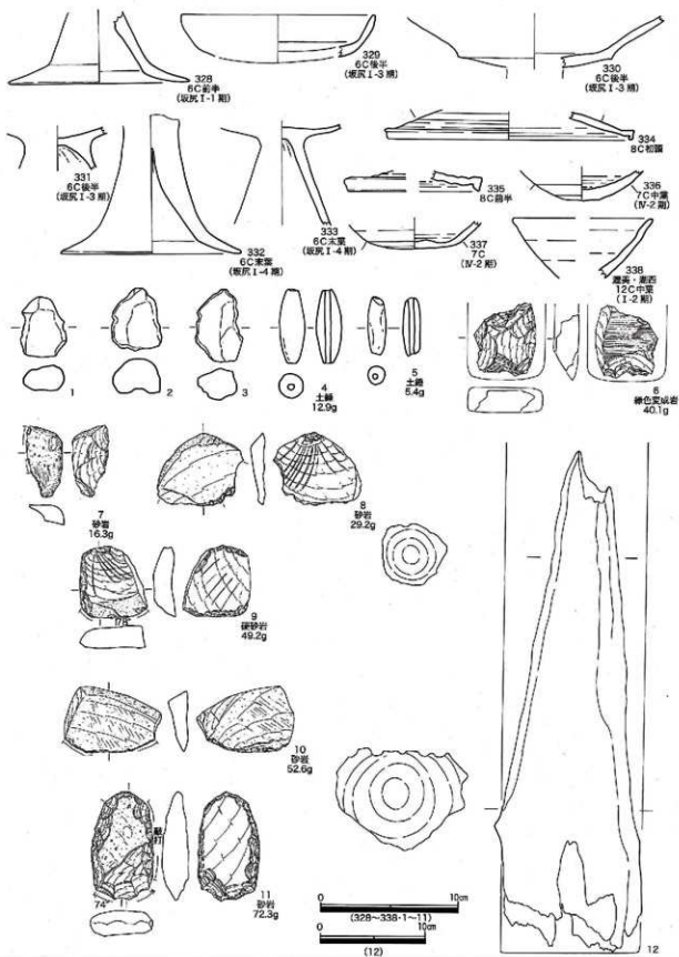
第101図 第62次 土器実測図12、土製品・石製品・木製品実測図
