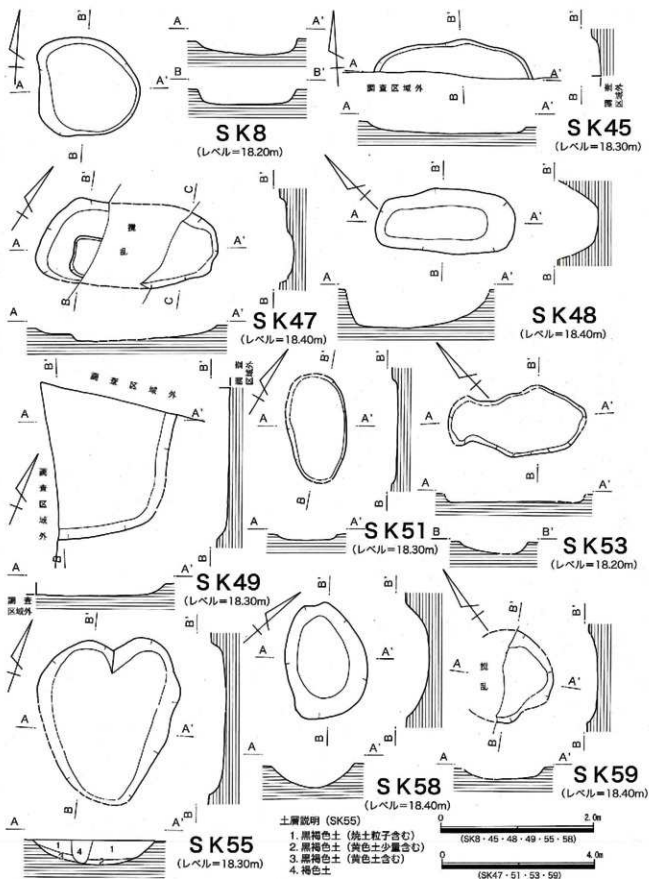
第108図 第63・75-1次 SK8・45・47～49・51・53・55・58・59実測図
