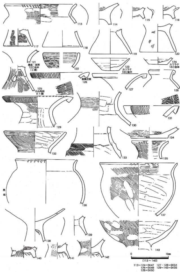
第115図 第63・75-1次 土器実測図5
