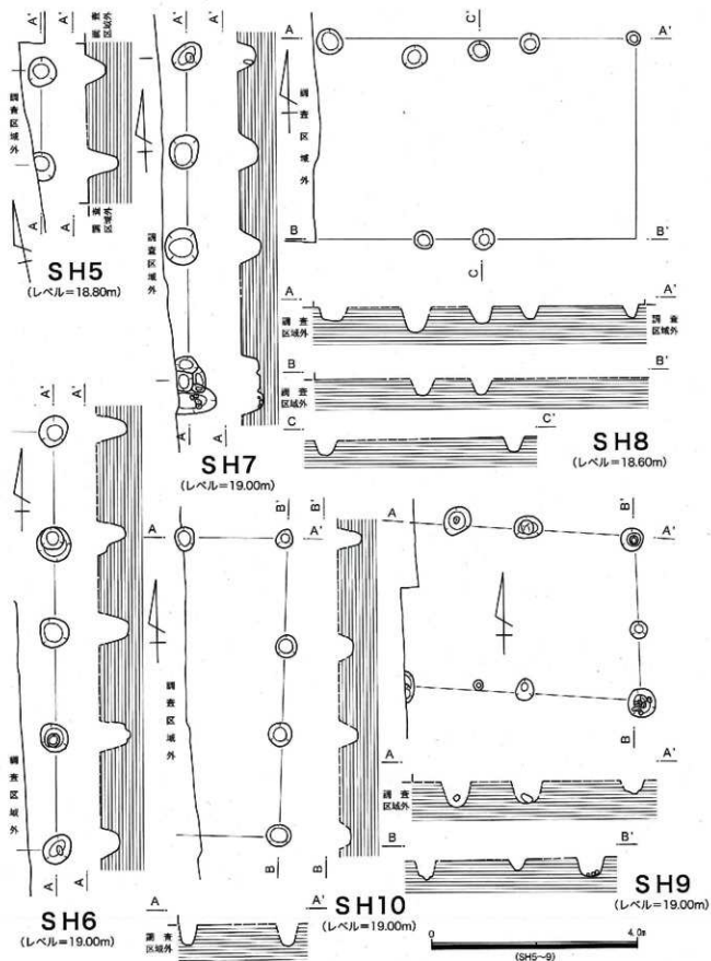
第87図 第62次 SH5～9実測図
