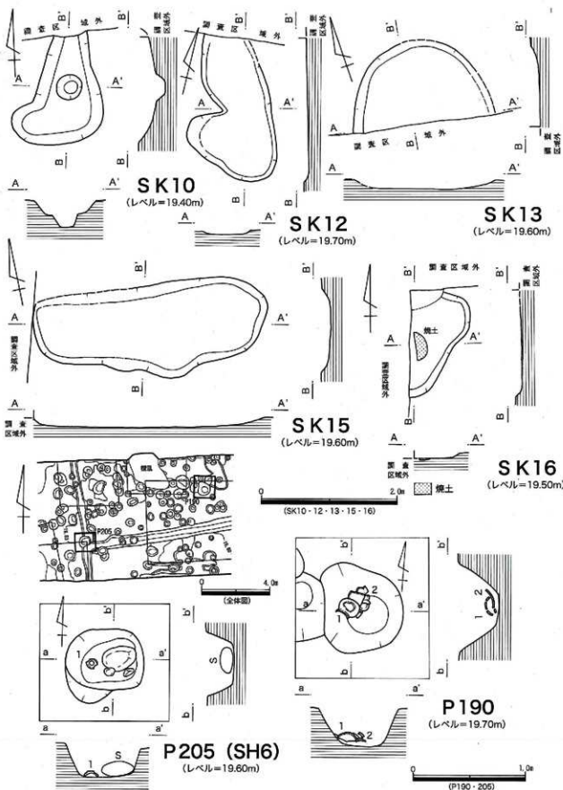
第29図 第59次 SK10・12・13・15・16、P190・205 (SH6) 実測図
