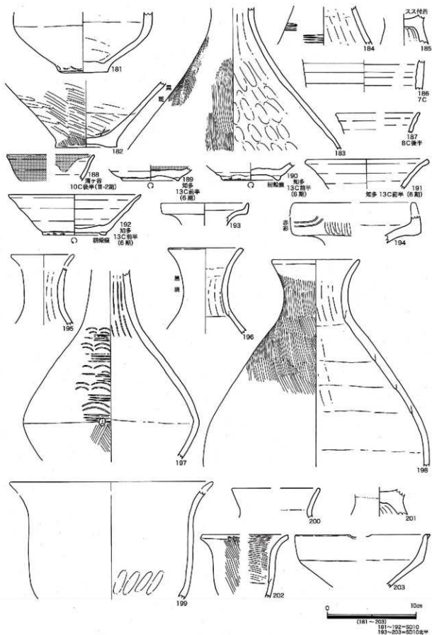
第68図 第61・72・74次 土器実測図6
