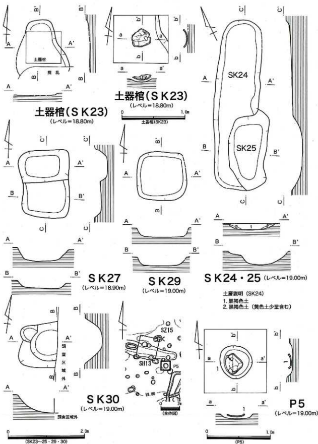
第9図 第57次土器棺 (SK23)・SK24・25・27・29・30、P5実測図s
