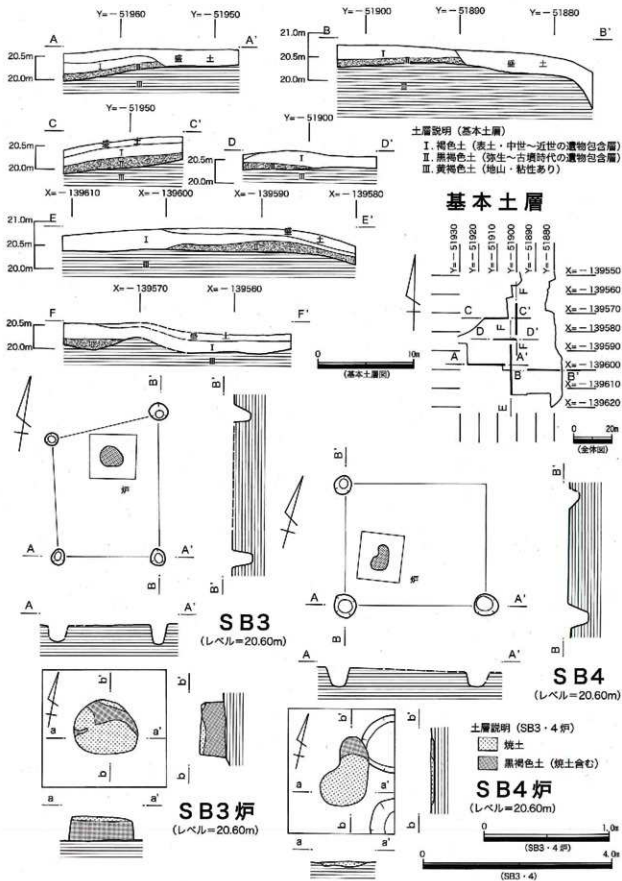
第50図 第61・72・74次 基本土層図、SB3・4実測図
