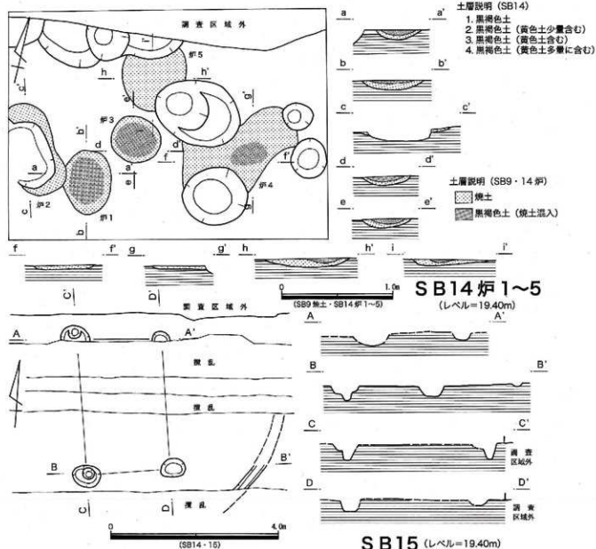
第16図 第58・77次 SB9 炉、SB14・15実測図
