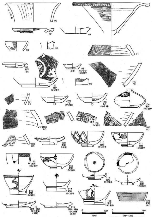
第132図 第47・51次 土器実測図4
