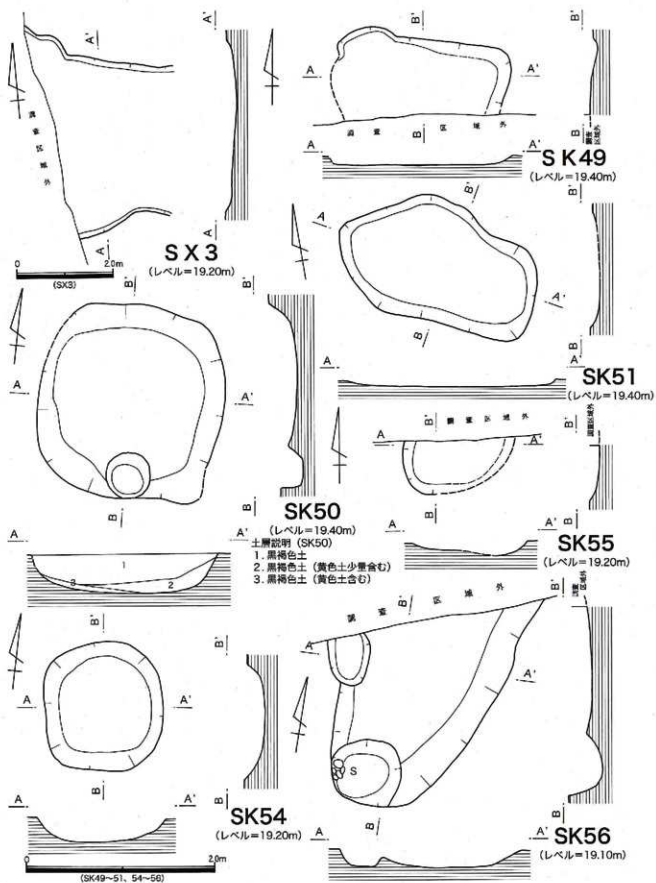
第174図 第52次 SX3、SK49～51・54～56実測図
