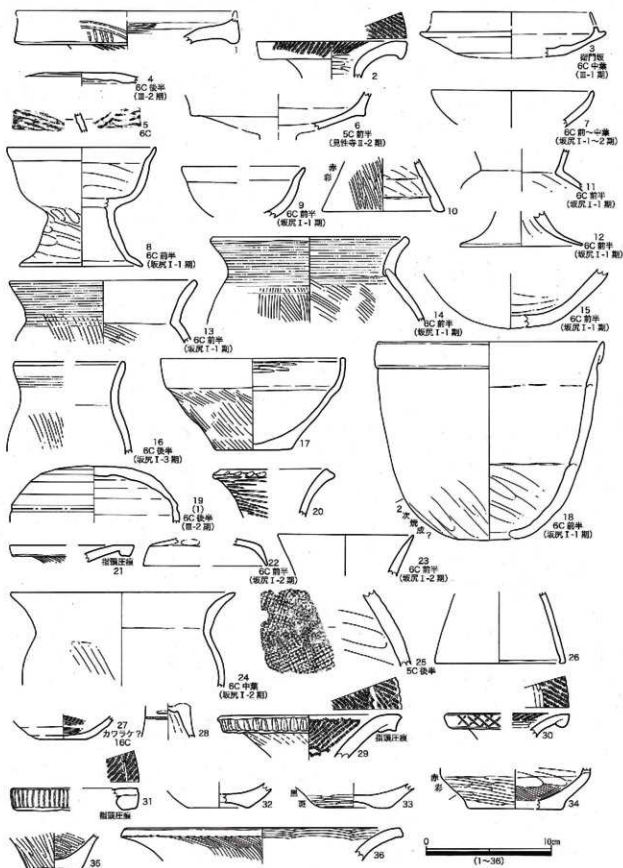
第164図 第50次 土器実測図1
