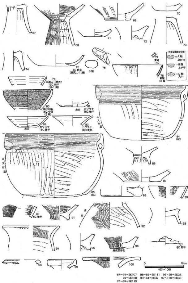
第166図 第50次 土器実測図3
