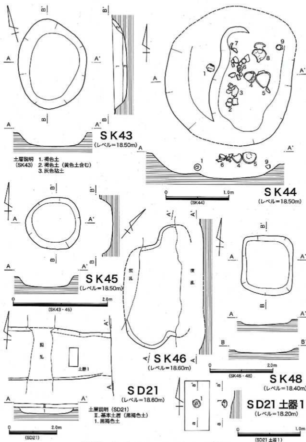
第197図 第54次 SK43～46・48、SD21実測図
