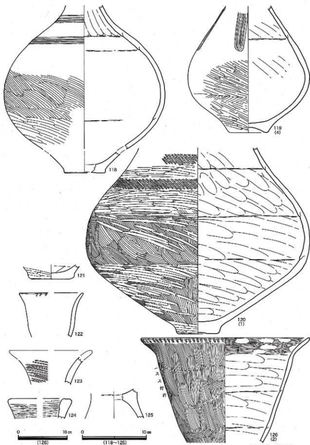
第218図 第55次 土器実測図5
