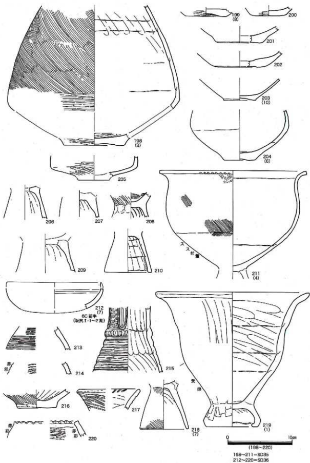
第156図 第49次 土器実測図9
