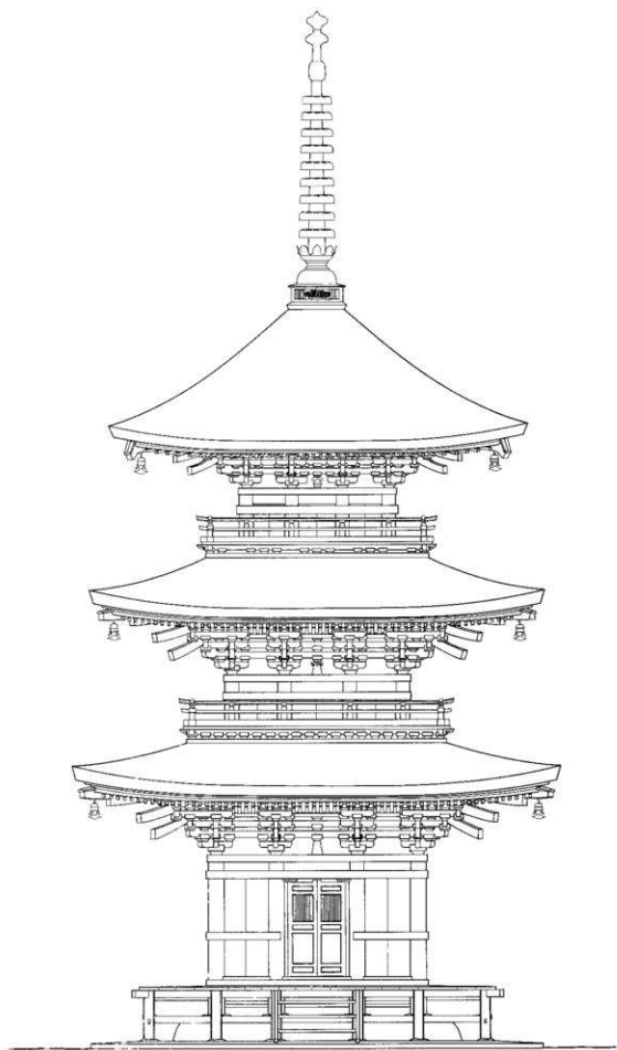
4 竣工立面图
