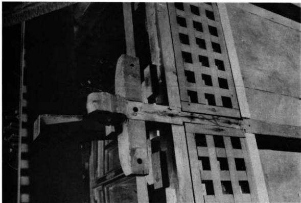
112 組立 軒天井、 秤肘木、 拳鼻の 取合せ
