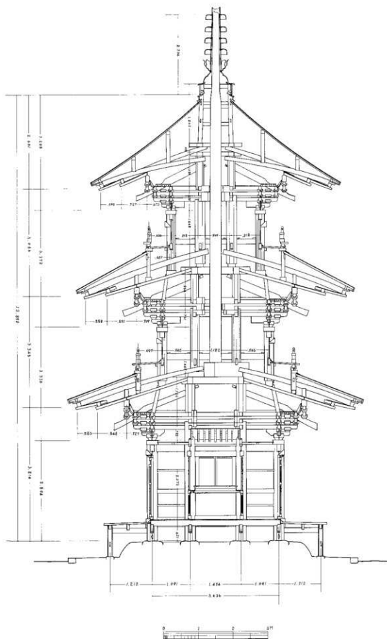
18 修理前 断面图
