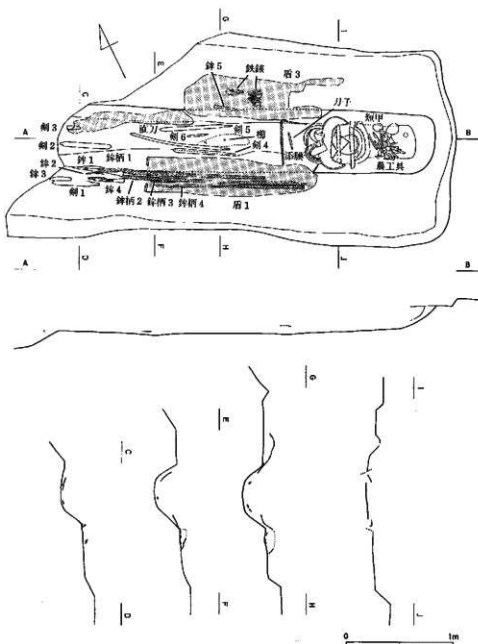
第4図 埋葬施設実測図
