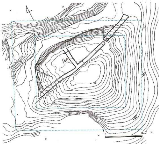
第2図 墳丘測量図 (調査前)
