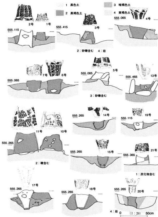
第15図 埋変断面実測図(1) (1~21号)
