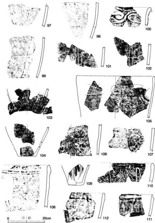
第27図 縄文土器実測図(11) (97~99: 2 住、100~102: 9 住、106・107: 6 住、103: 45 埋、104: 41 埋)
