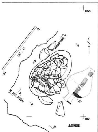
第13圖 遺構実測図(11) (D62~64・74・84・94周辺、土器棺墓)
