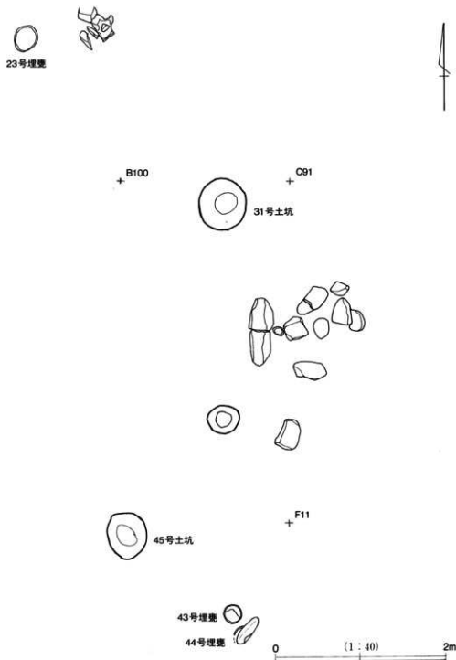
第8图 遺構実測図(6) (B100、C91、E10・20・30、F1・11・21周辺)
