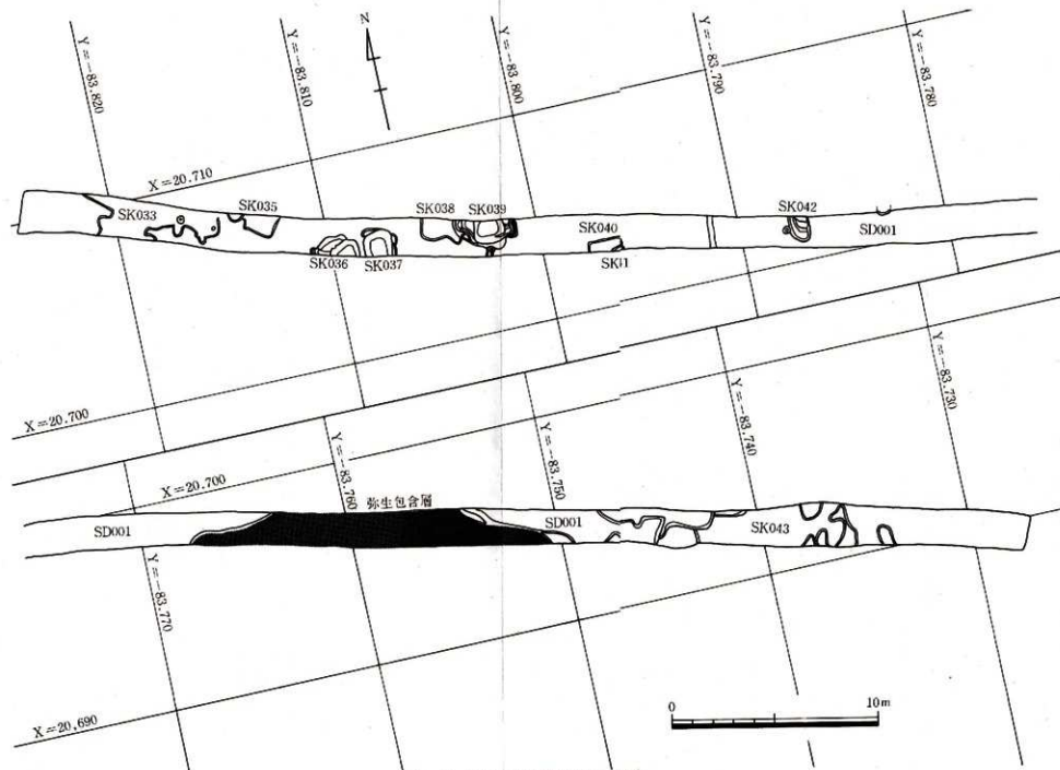
Fig. 13 B地区遺構配置図 (S=100)
