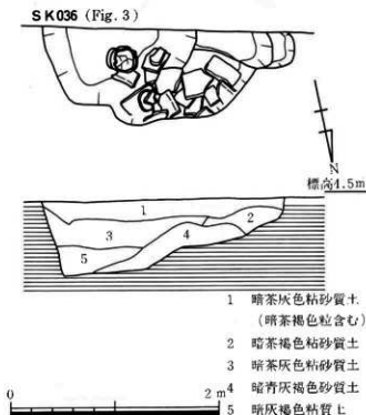
Fig. 3 SK036実測図 (S=1/40)
