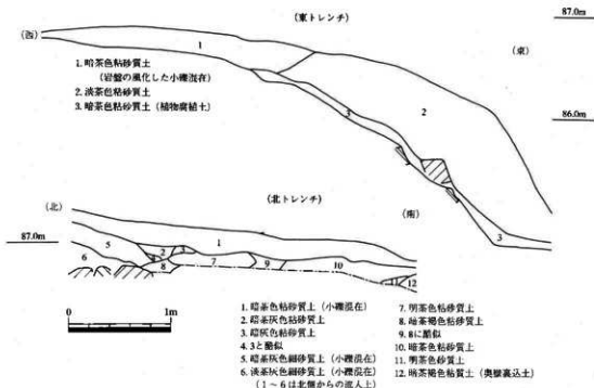
Fig. 3 東西・南北土層断面図 (S=1/40)
