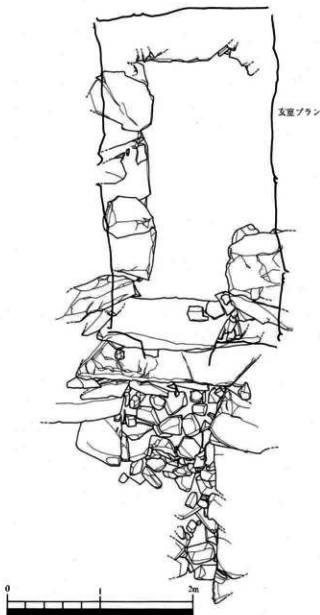
Fig. 4 玄室上面・羨道実測図 (S=1/40)
