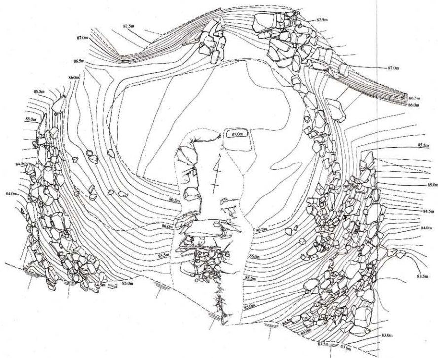
Fig.12 填丘・葦石実測図 (S=1/60)
