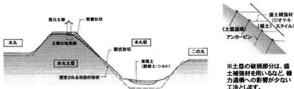
本丸土塁整備模式図
