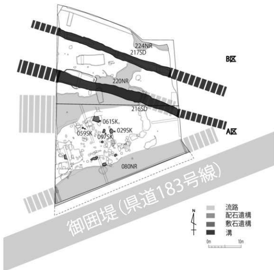
主要遺構配置図(S=1/400)
