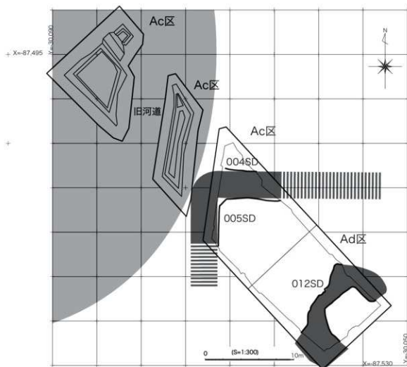
23A 区全体図
