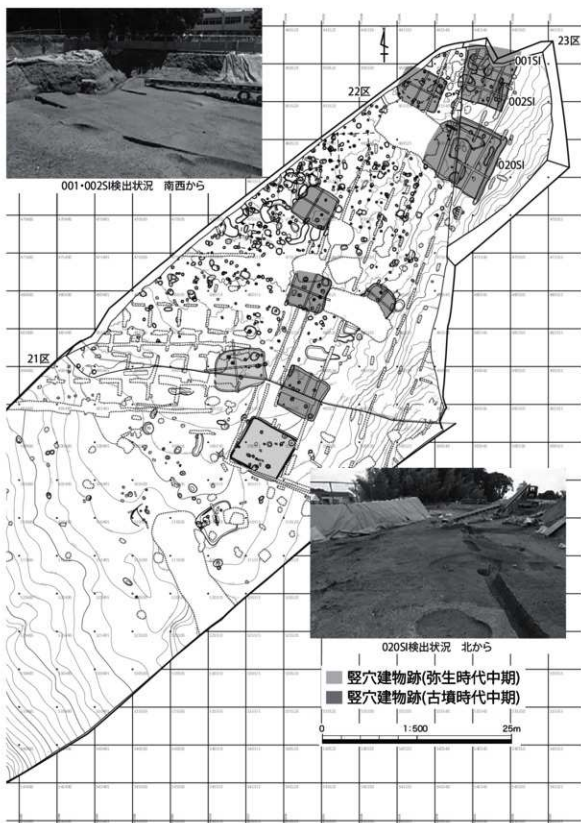
遺構全体図 (S=1/500)
