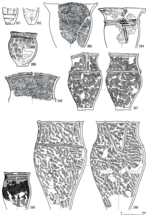
図VII-27 H-8 土器261~269
