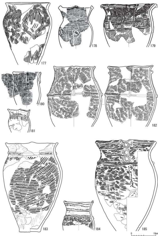
図VII-19 H-3 土器177~185
