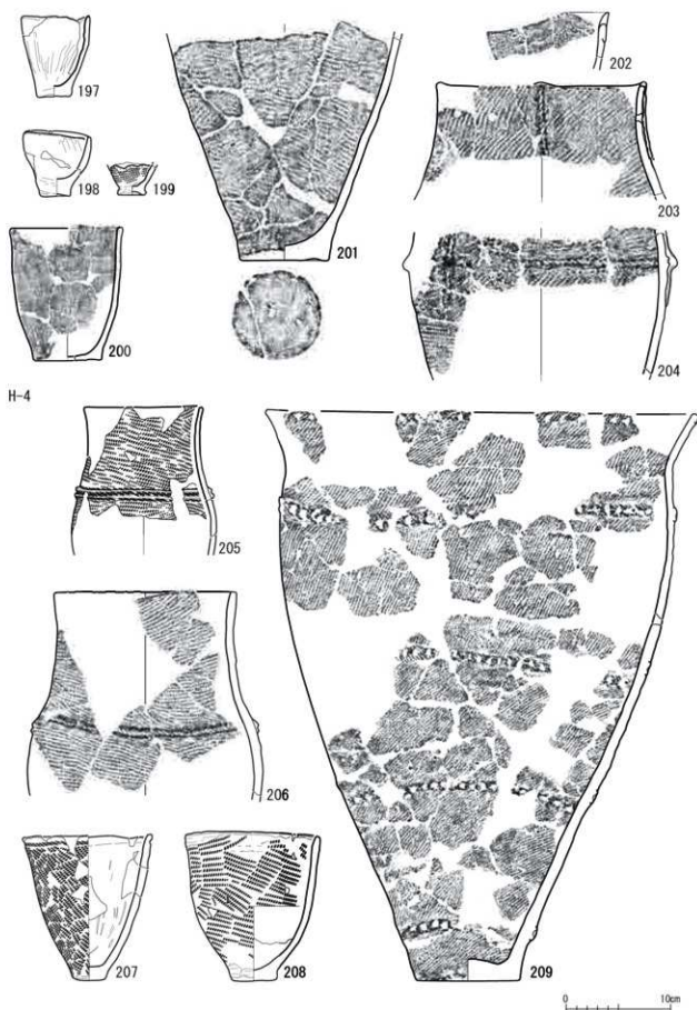
図VII-21 H-3・4 土器197~209
