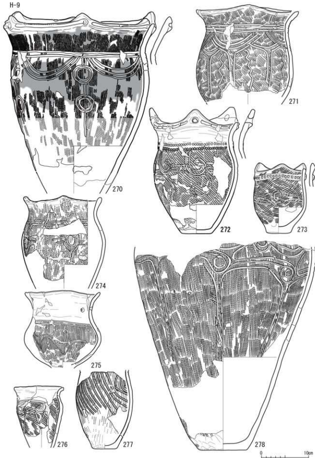
図VII-28 H-9 土器270~278
