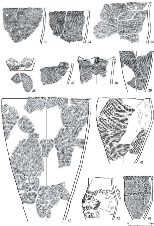
図VII-5 H-1 土器33~43
