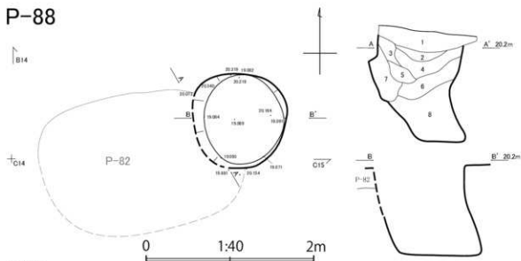
P-88 A-A'
