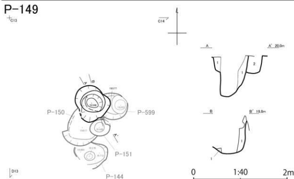
P-149 A-A'
