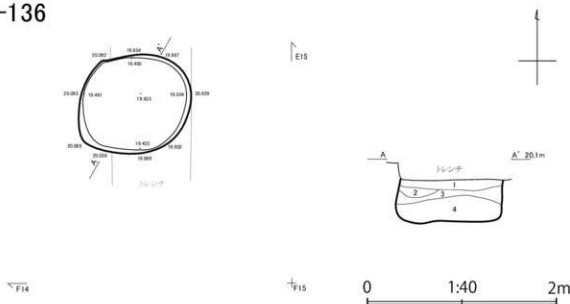
P-136 A-A'
