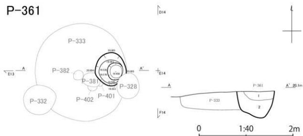
P-361 A-A'
