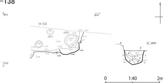
P-138 A-A'
