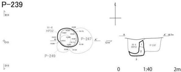
P-239 A-A'
