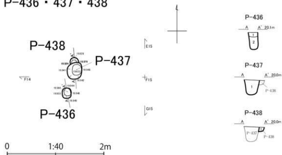
P-436 A-A'
