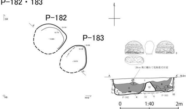
P-182・183 A-A'
