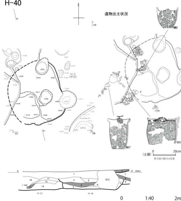
H-40 A-A'
