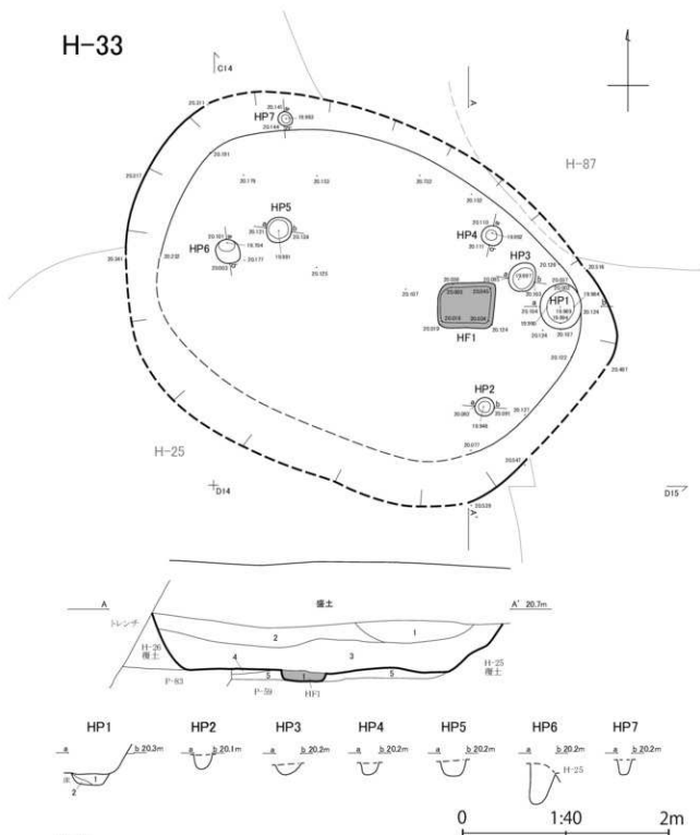
H-33 A-A'
