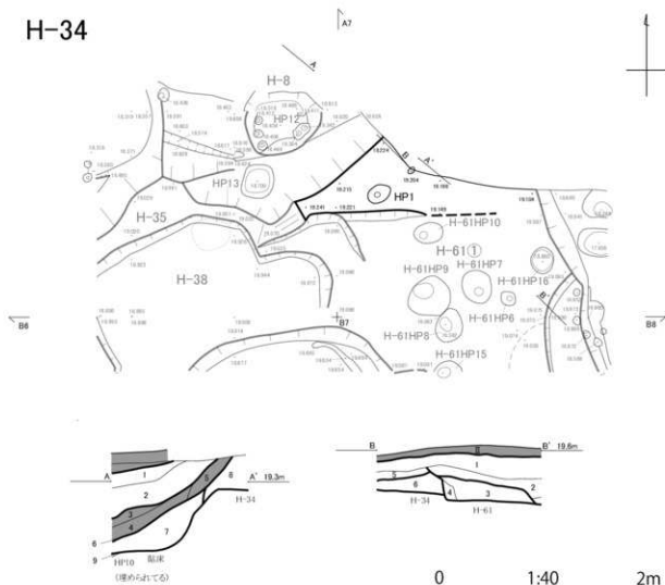
H-34 A-A'
