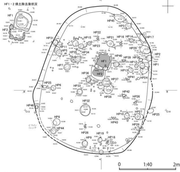
住居変遷図
