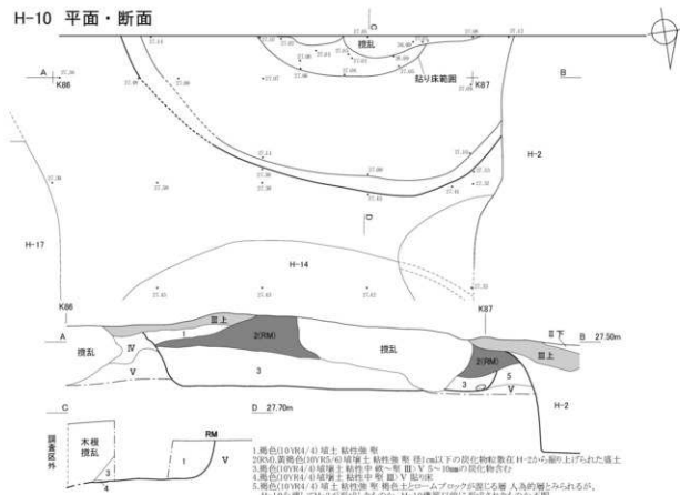
遺物分布
