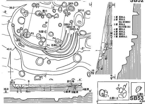
第27図 S B51~53実測図
