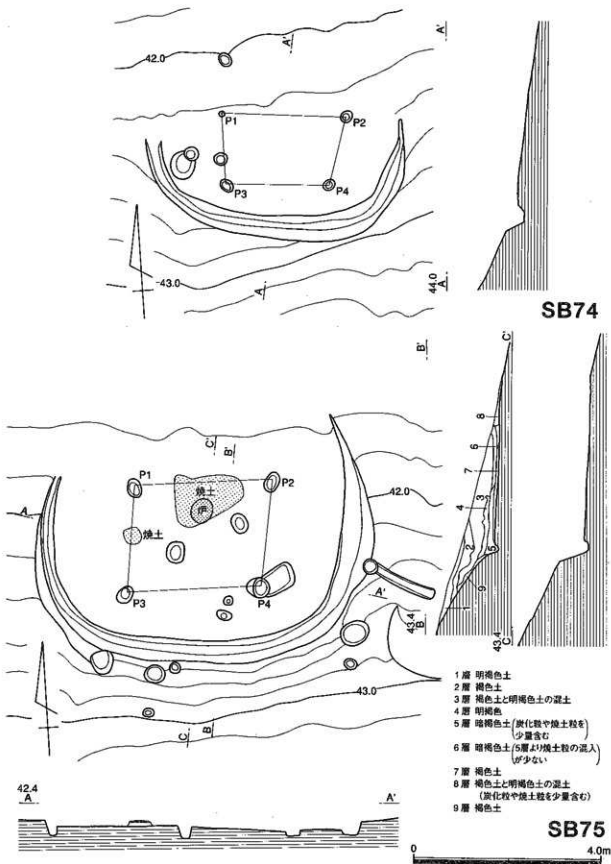
第37図 S B 74・75実測図
