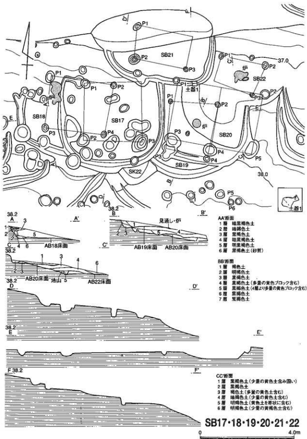
第16図 SB17~22実測図
