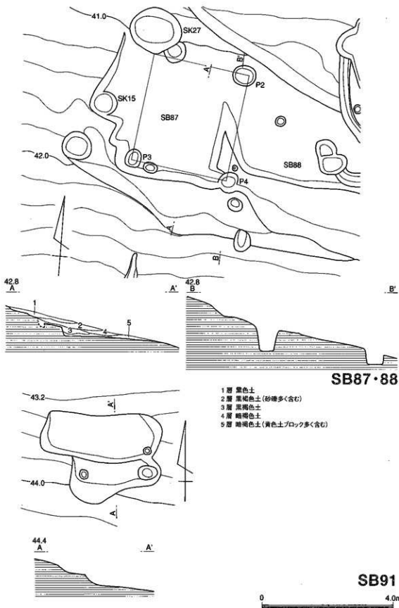
第41図 S B 87・88・91実測図
