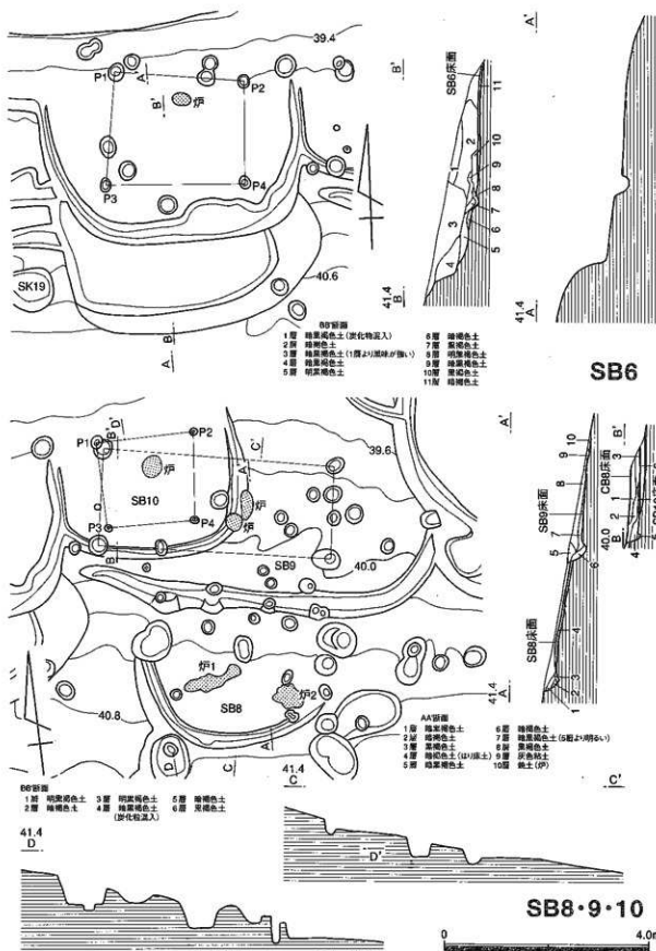
第11圖 SB 6・8～10実測図
