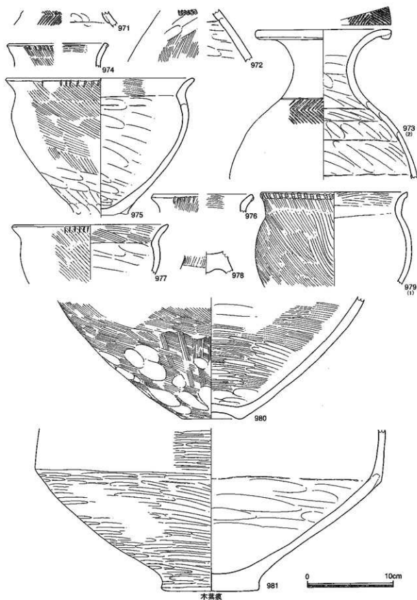
第158图 土器実測図31
