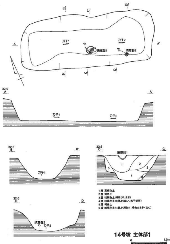
第126図 B 14号墳主体部1 実測図
