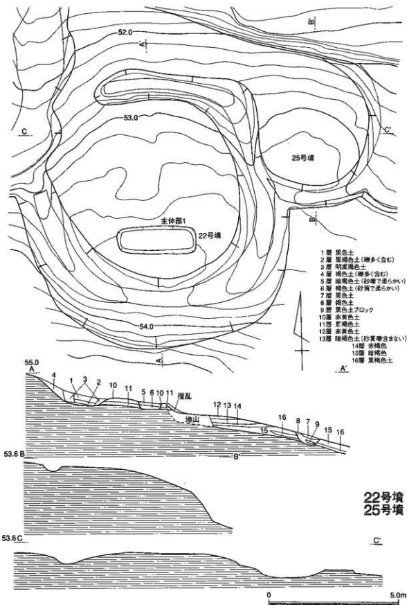
第90図 B 22・25号墳実測図
