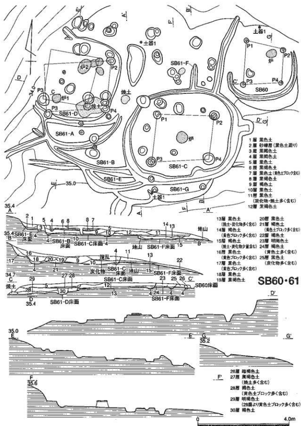
第31図 S B 60・61実測図
