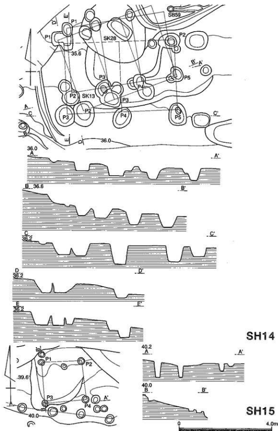
第51圖 SH14・15実測図
