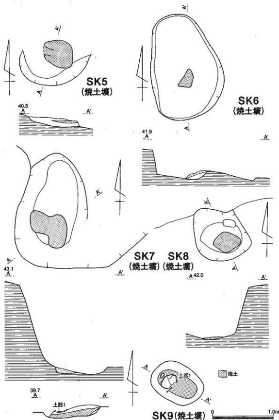
第80図 SK5～9 実測図
