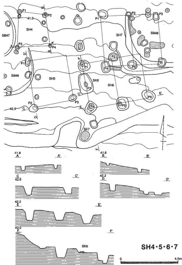
第49図 SH4~7実測図
