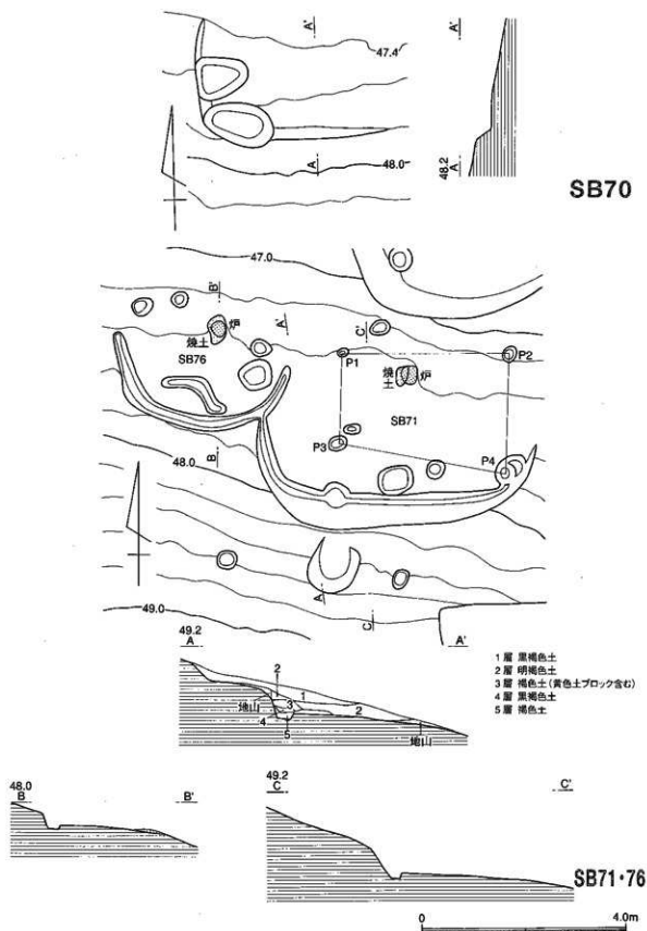
第35図 S B 70・71・76実測図
