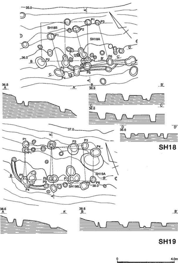
第53図 SH18・19実測図
