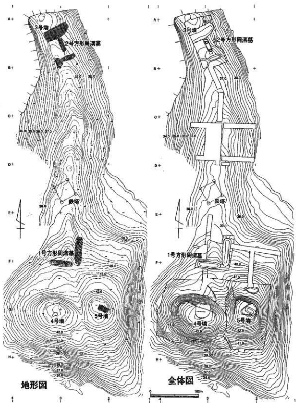
第4图 A地区地形・全体图
