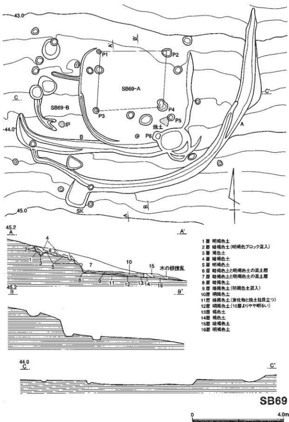
第34図 S B 69実測図
