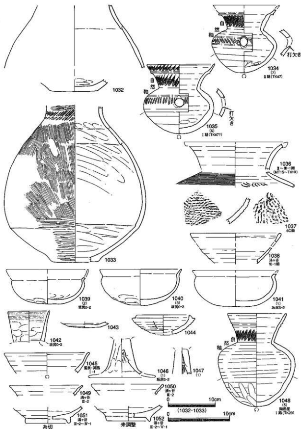
第161圖 土器実測図34
