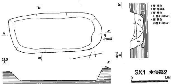
第111図 3号方形周溝墓 主体部2 SX1主体部1・2 実測図
