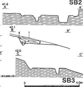
第10図 SB2・3実測図
