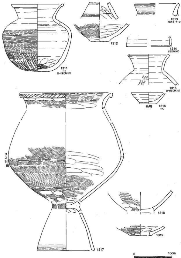
第174図 土器実測図47
