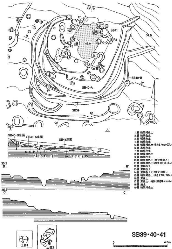
第22図 S B39~41実測図
