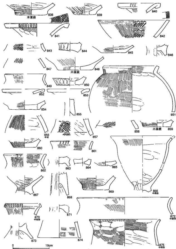
第154圖 土器実測図27
