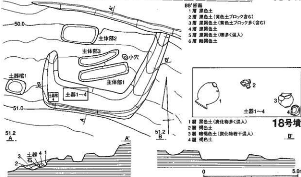
第86図 B 15・18号墳実測図
