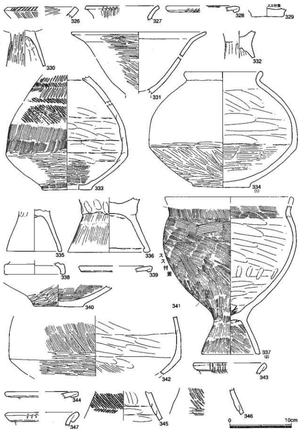
第137図 土器実測図10
