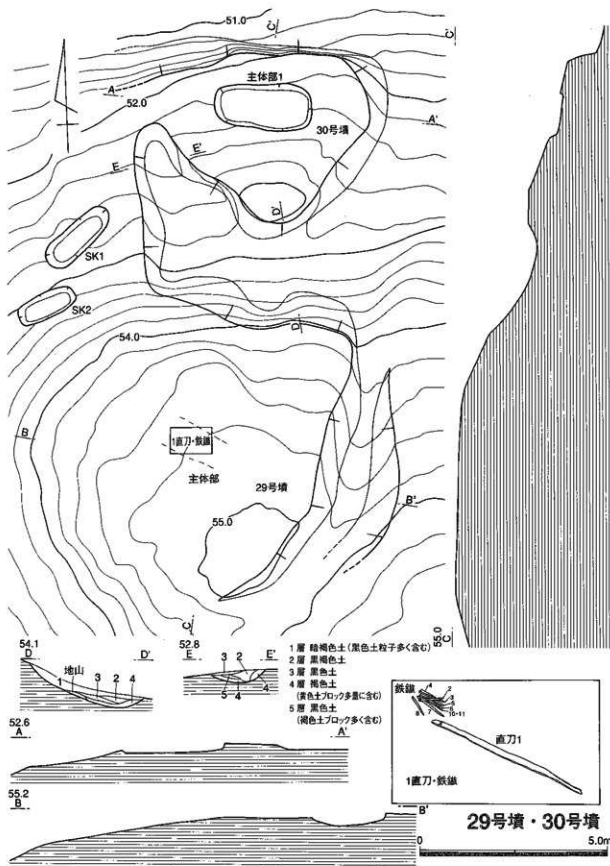
第93図 B 29・30号墳実測図
