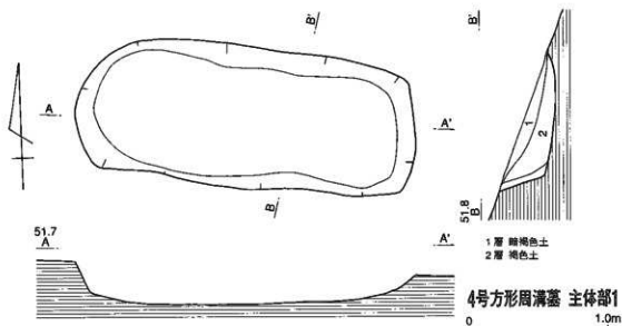
第74図 3・4号方形周溝墓主体部実測図
