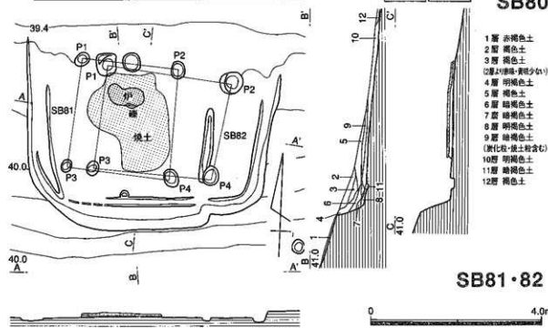
第39図 S B 80~82実測図
