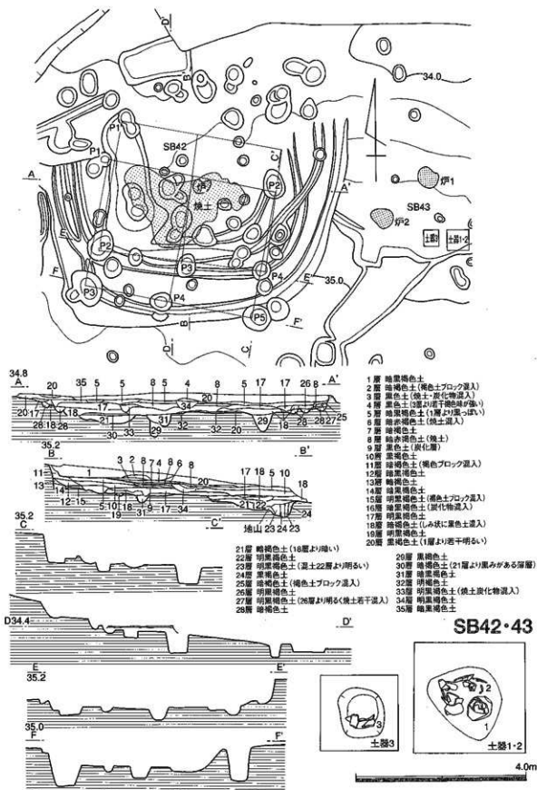
第23図 S B42・43実測図
