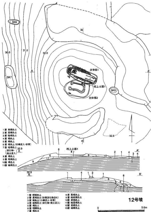
第119図 B 12号墳実測図
