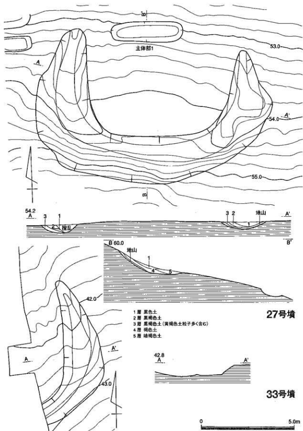
第92図 B 27・33号墳実測図
