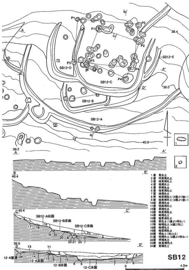
第14図 SB12実測図
