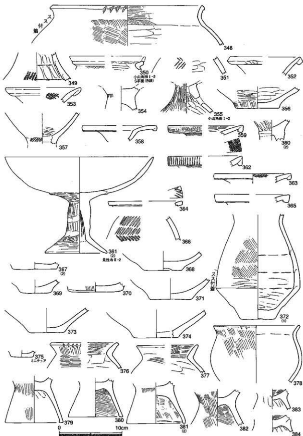
第138図 土器実測図11
