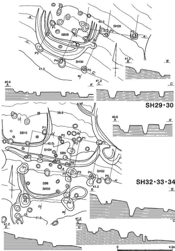
第57図 SH29・30・32~34実測図
