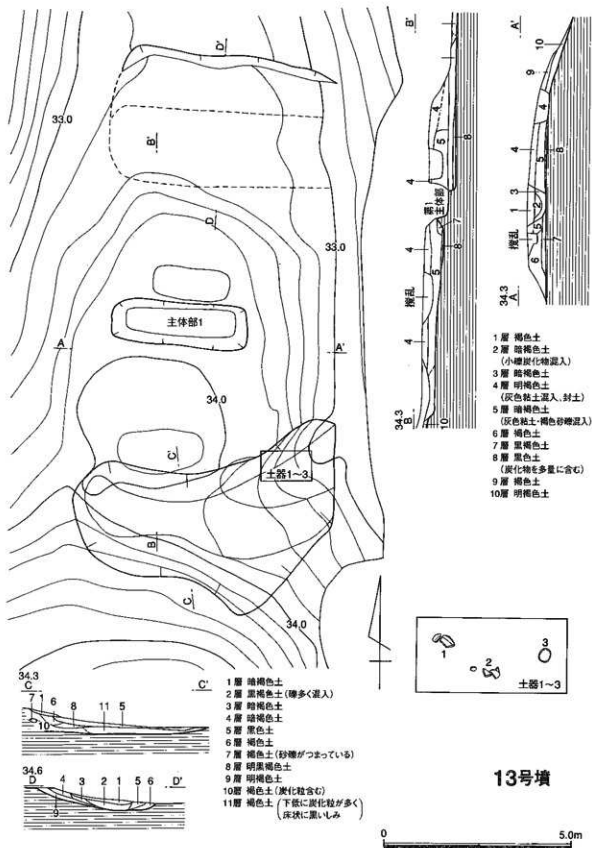
第120図 B 13号墳実測図
