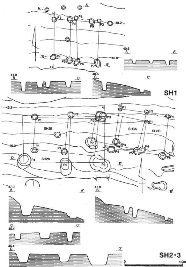
第48図 SH1~3実測図
