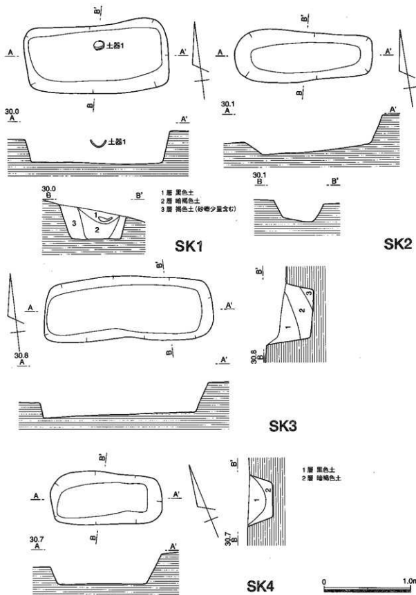
第114圖 SK 1~4 実測図
