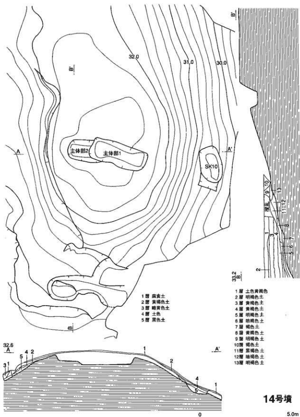
第121图 B 14号墳实测图
