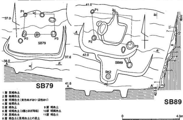
第38図 S B 78・79・86・89実測図
