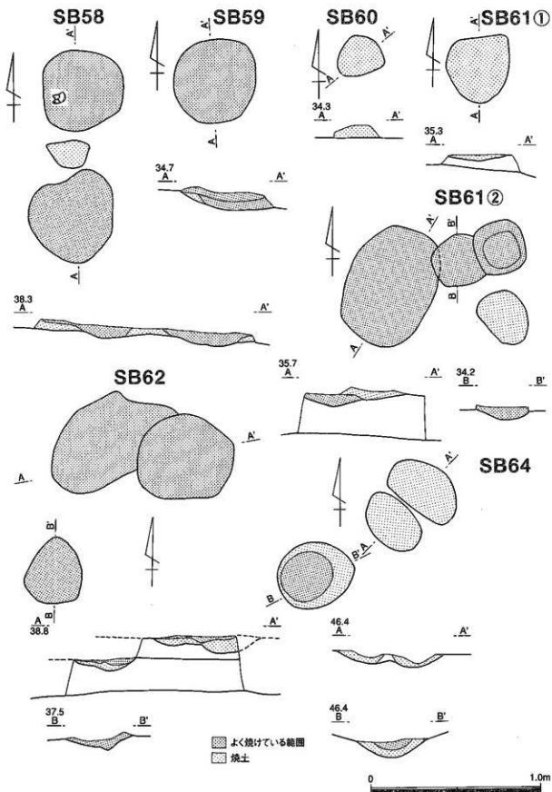
第46図 S B 58~62・64炉実測図
