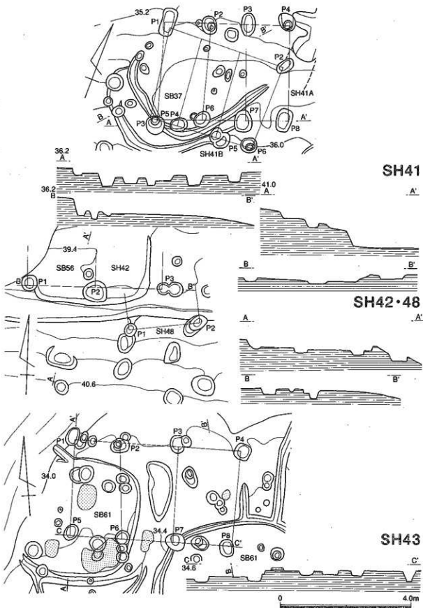
第60圖 SH41~43・48実測図
