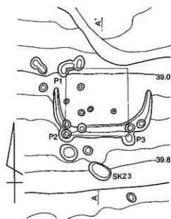
第13図 SB11・13実測図
