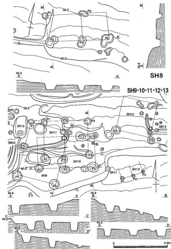
第50図 SH8~13実測図
