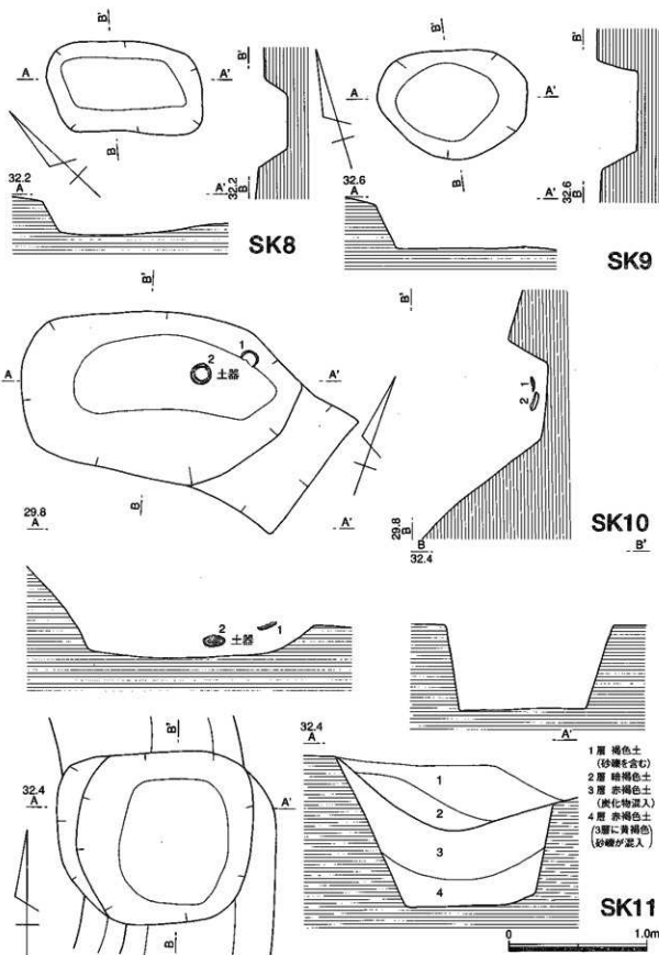
第116図 SK8～11実測図
