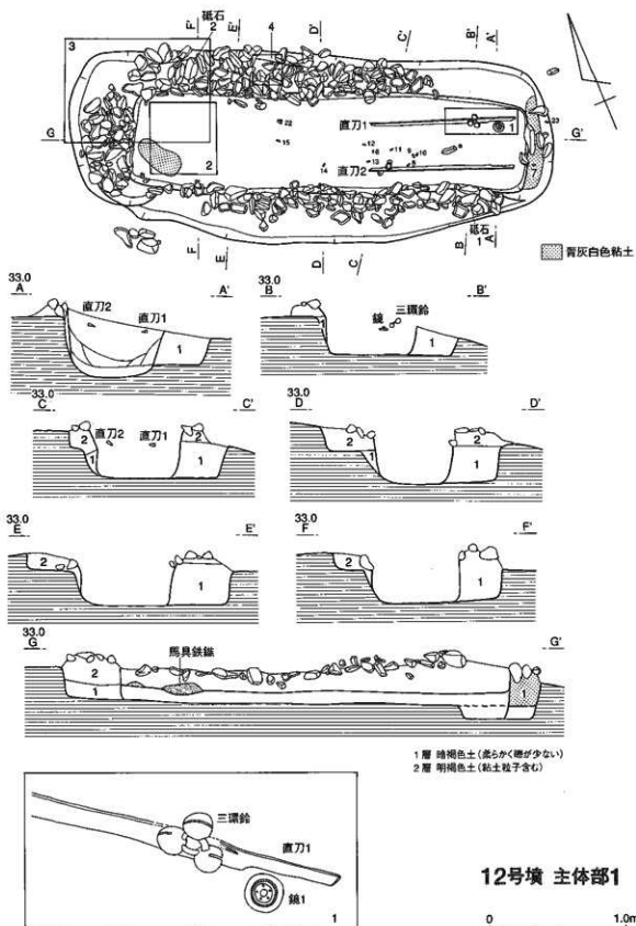
第123図 B12号墳主体部1 実測図
