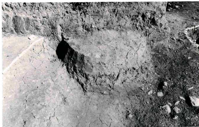
(2) SB 3 かまど (芯材と思われる砂質の粘土、部分的に焼土塊が見られる。西より)
