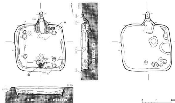
1. M38-S112 実測図 (1/80)
