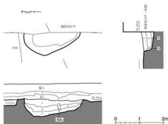
1. M37-SX 17 実測図 (1/80)
