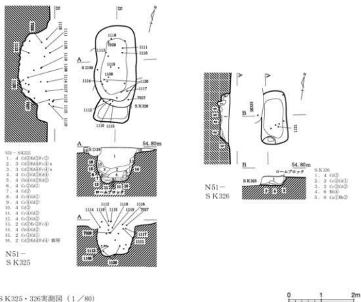
1. N51-S K325・326実測図 (1/80)
