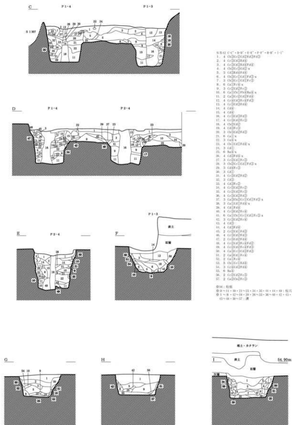
1. N51-SB42断面実測図 (1/40)
