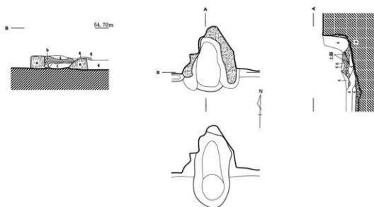
3. N51-S1303掘実測図 (1/40)
