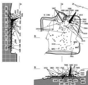
1. N51-S 1301実測図 (1/80)
