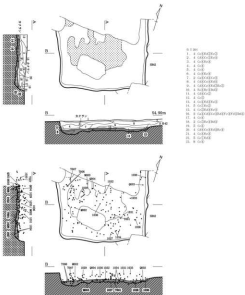
1. N51-S1304実測図 (1/80)
