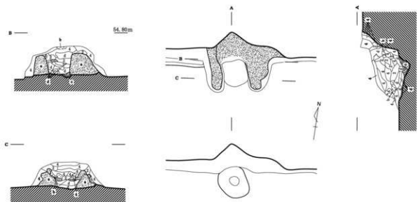
1. N51-S1307実測図 (1/40)
