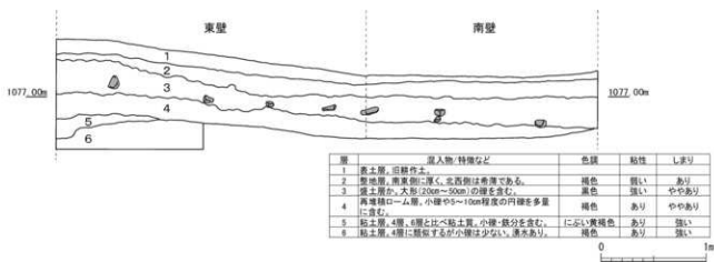
第7図 土層断面図 (S=1/40)
