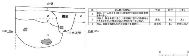
第4図 土層断面図 (S=1/40)
