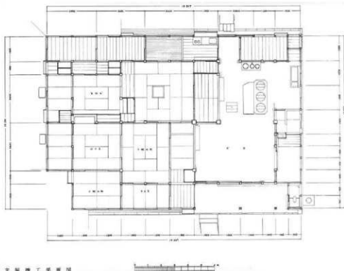
図 4-5 大塚家住宅平面図
