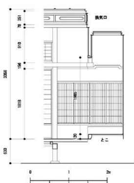
図 3-13 奥座敷床詳細図（作図：設計集団 LN）
