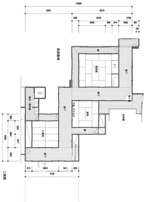
二階廊及び奥座敷棟一階平面図
