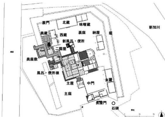
図 2-2 旧山崎家住宅配置図（現況）
