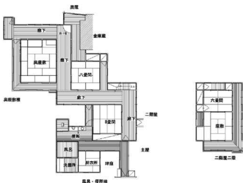
圖 3-12 奥座敷棟、二階屋、風呂・便所棟室名
