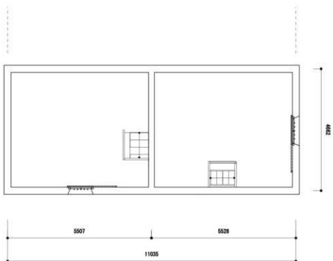
西藏2阶平面图
