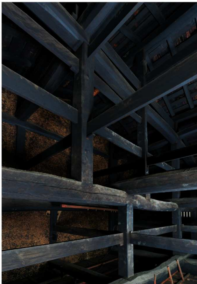
5. 主屋 土間側小屋組（南東より）
