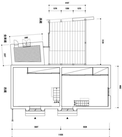
奥藏·西藏·金库藏1阶平面图
