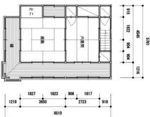
二階廊二階平面図
