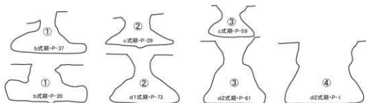
図 VI-1 フラスコ状土坑の断面形状
