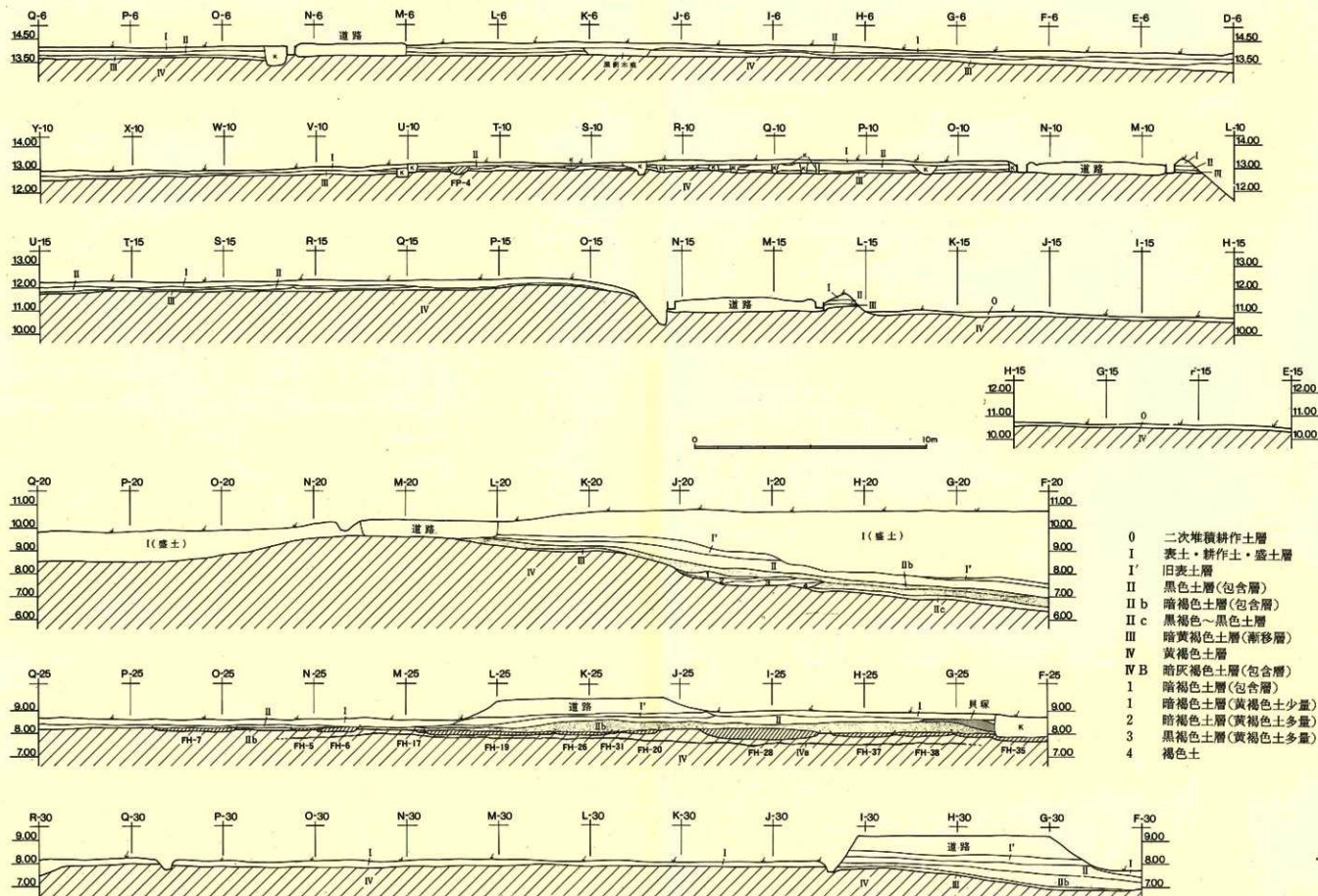
图II—9 道路土層断面图(2)
