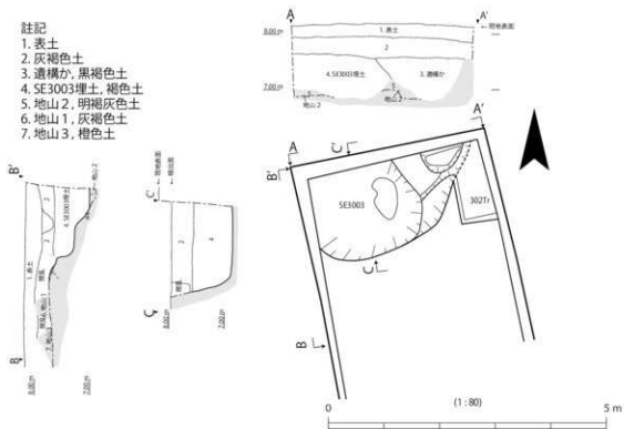
第18図 井戸SE3003 平面図・断面図
