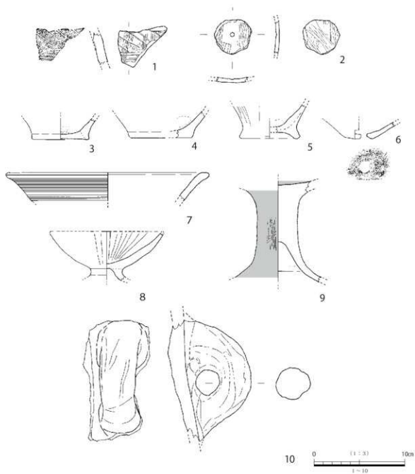
第16図 溝SD3001最下層3層 遺物実測図(3)
