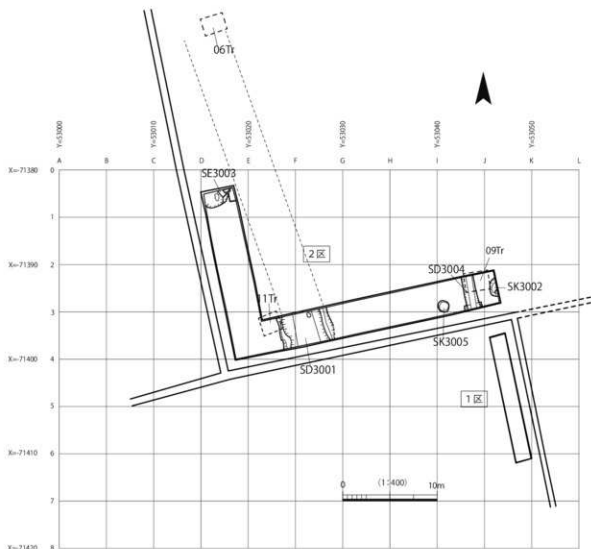
第4図 遺構配置図
