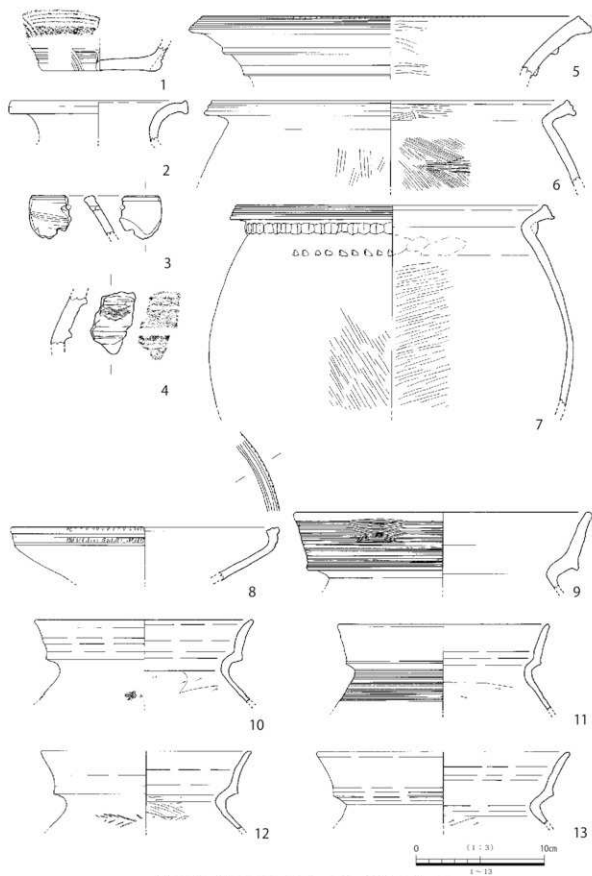
第15図 溝SD3001 最下層3層 遺物実測図(2)
