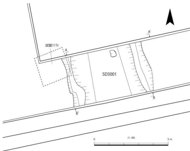
第6図 溝 SD3001 遺構平面図
