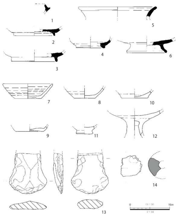
第9図 溝SD3001下層 遺物実測図
