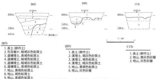
第5図 試掘トレンチ (北壁) 断面図 (S = 1 : 80)
