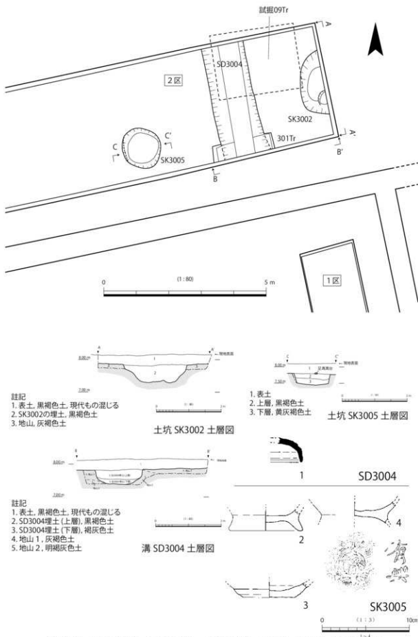
第20図 土坑 SK3002・溝 SD3004・土坑 SK3005 平面図・断面図・遺物実測図
