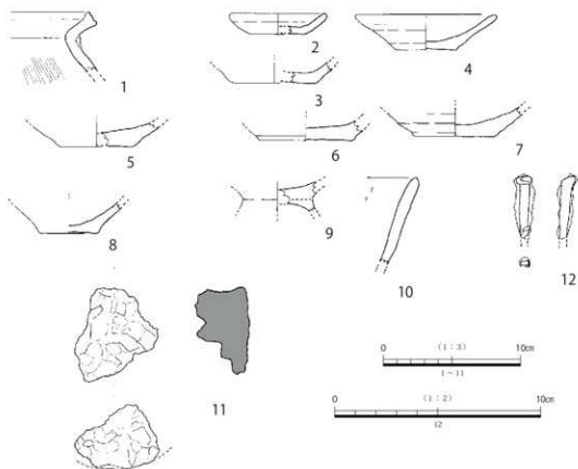
第19図 井戸SE3003 遺物実測図
