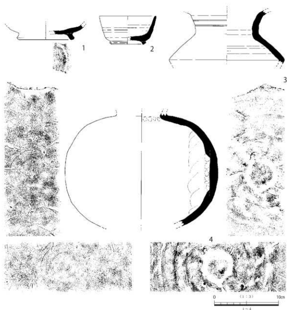
第13図 溝SD3001 最下層3層 遺物実測図(1)
