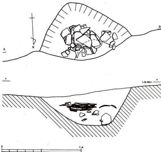
第6図 入来遺跡Bトレンチ土坑図
