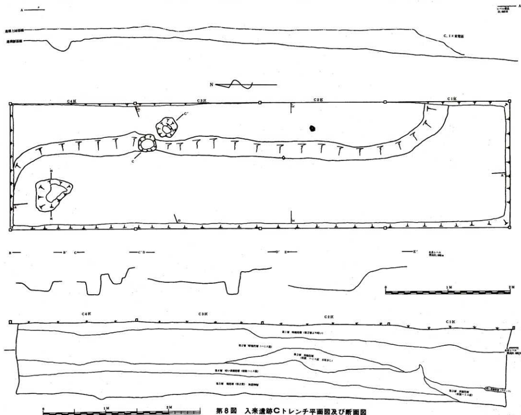
第8図 入来遺跡Cトレンチ平面図及び断面図
