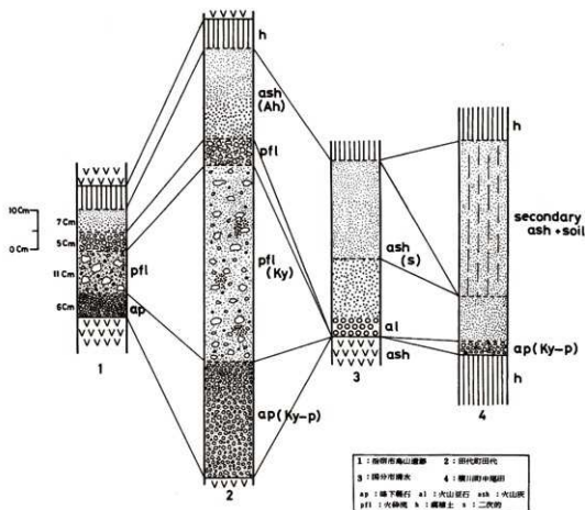
図11 アカホヤの対比
