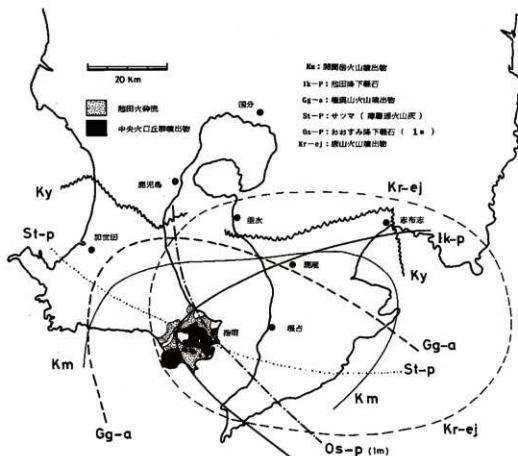
図13 指宿地方でみられる火山噴出物の分布範囲
