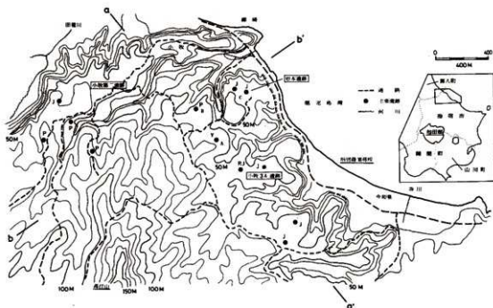
図5 北部台地等高線図
