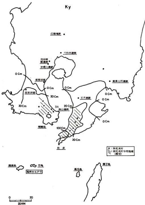
図10 アカホヤ（幸屋火砕流）中の火砕流部分の分布 及び炭化木の存在する地点（分布は平井による）
