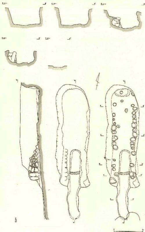
第10図 三沢2号墳 主体部
