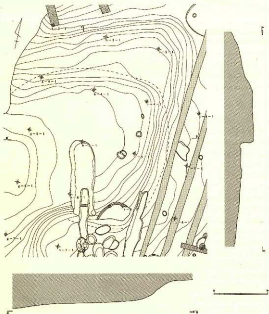
第9図 三沢2号墳
