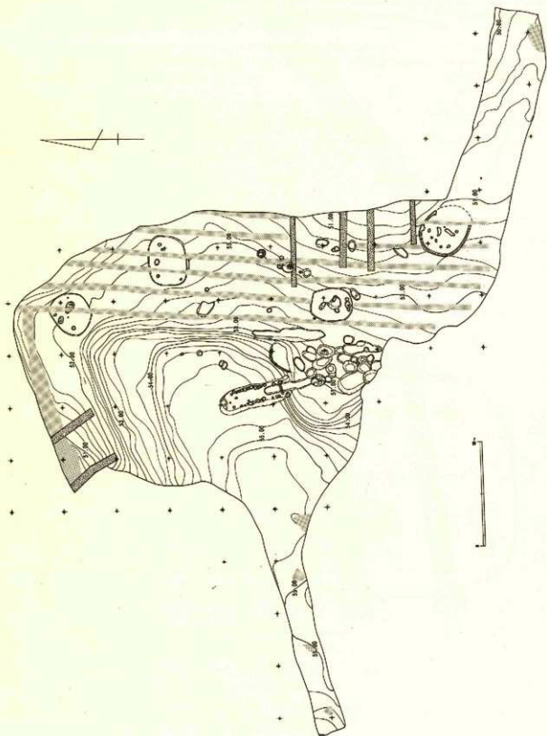
第3図 全体図
