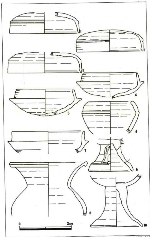
▲出土遺物実測図(2)
