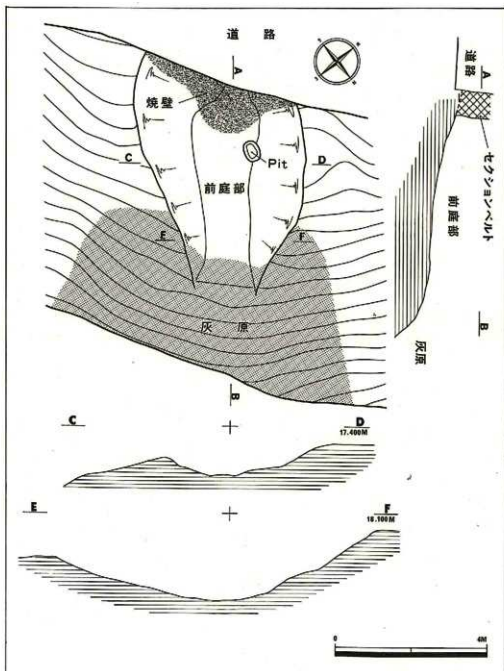
▲ 3号竈跡前庭部実測図
