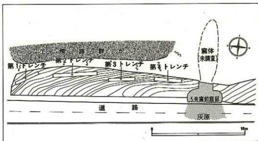
▲南門坂古窯南地区実測図
