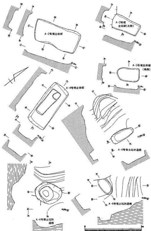
第7図 愛野向山A-2・3・4号墳主体部・土状遺構実測図
