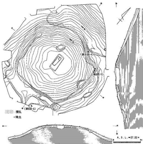
第6図 愛野向山A—4号墳実測図
