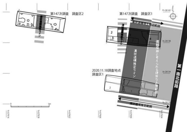
第 18 図 町 147 次各施設分布イメージ図 (1 : 150)
