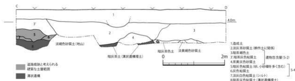
第16図 調査区1 遺構配置図・土層図(1/100・1/60)
