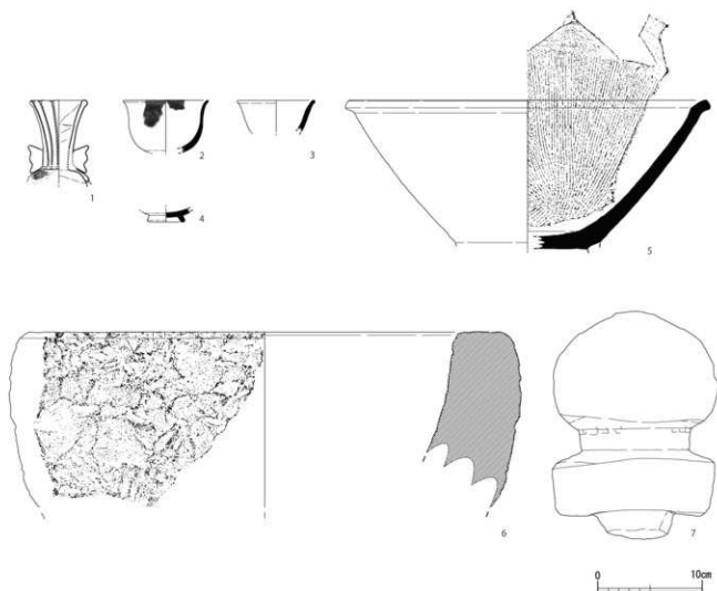
第23図 SK065出土遺物実測図1(1/4)
