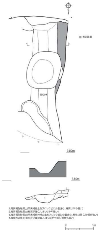
第 16 図 SF099 遺構実測図 (1/40)
