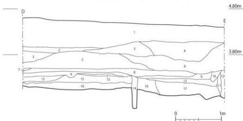
第8図 調査区南壁(C-D間)土層断面図(1/40)
