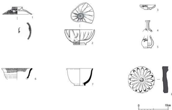
第 27 図 SD146 出土遺物実測図 5 (1/4)
