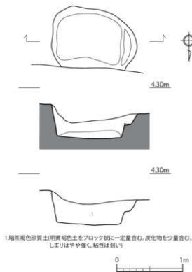
第10図 SK065 遺構実測図(1/40)
