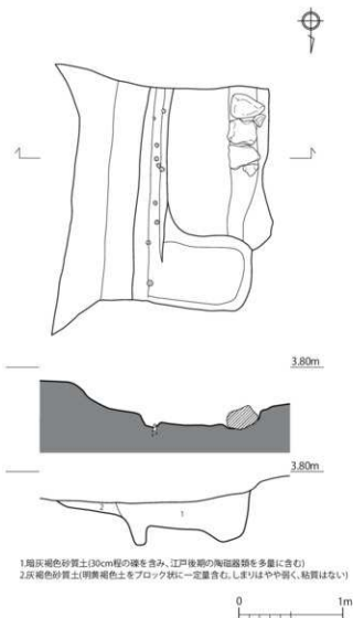
第 15 図 SD146 遺構実測図 (1/40)
