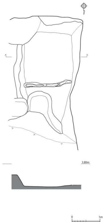
第 22 図 SF210 遺構実測図 (完掘時)(1/40)
