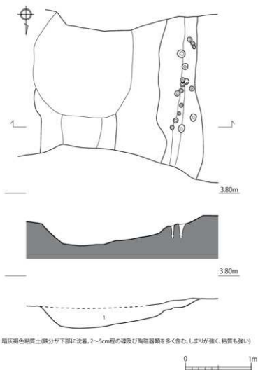
第14図 SD14S 遺構実測図(1/40)
