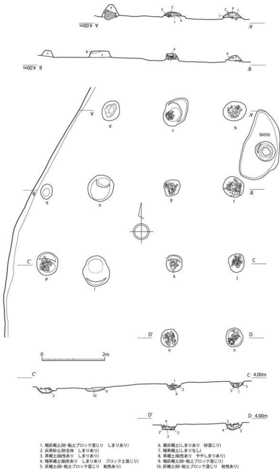
第10図 SB065 遺構実測図 (1/60)
