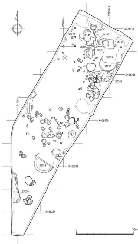
第 28 図 第 3 面 全体遺構図 (1/200)
