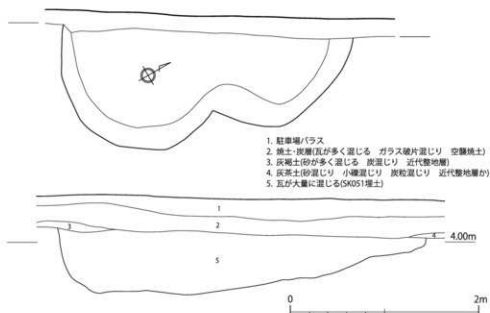
第 23 図 SK051 遺構実測図 (1/40)
