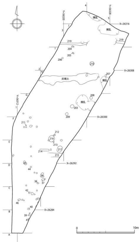
第 36 図 第 4 面遺構配置図 (1/200)
