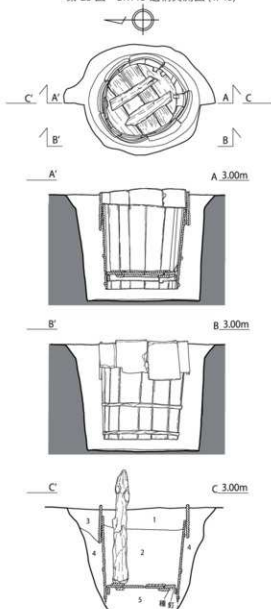
第 25 図 SK115 遺構実測図 (1/40)
