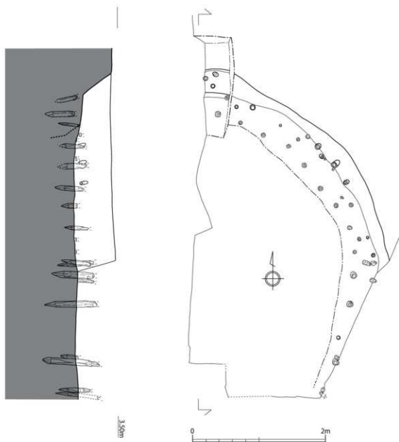
第14図 SG010 古段階遺構実測図 (1/40)
