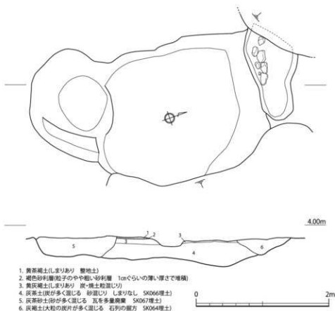
第 24 図 SK066・SK067 遺構実測図 (1/40)
