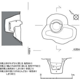
第16図 SK015 遺構実測図 (1/30)
