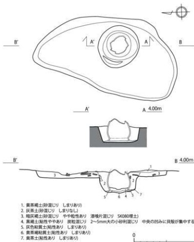
第17図 SK050 遺構実測図 (1/30)
