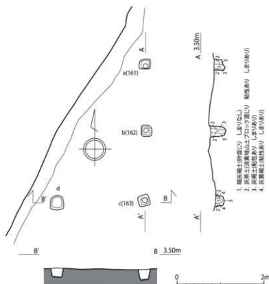
第 29 図 SB220 遺構実測図 (1/60)
