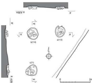
第 13 図 SB218 遺構実測図 (1/60)
