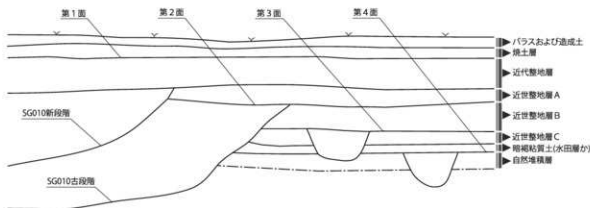
第3図 土層模式図
