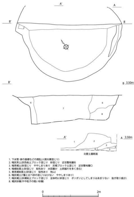
第30図 SE033 遺構実測図(1/40)
