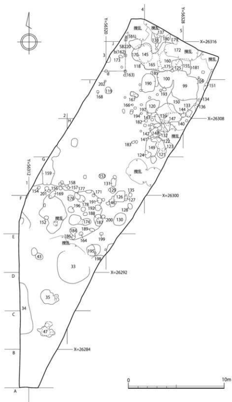
第27図 第3面遠構配置図 (1/200)
