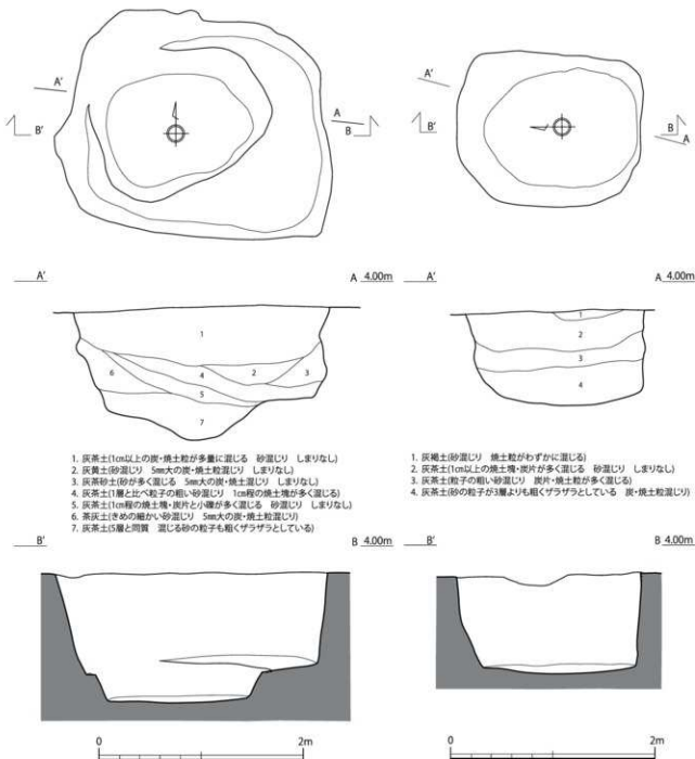
第 18 図 SK099 遺構実測図 (1/40)
