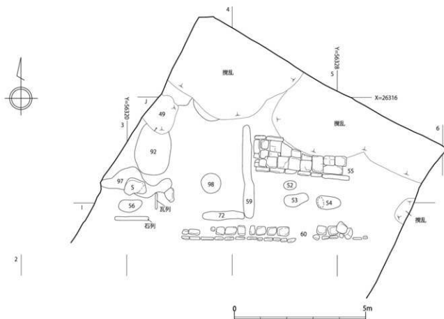
第6図 第1面 遺構配置図(1/100)
