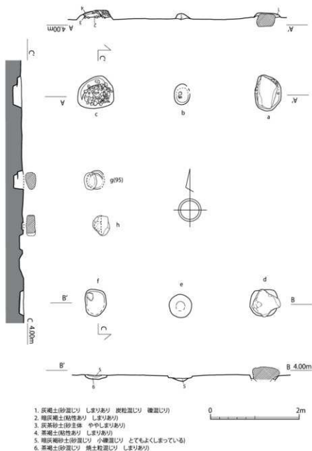
第 11 図 SB070 遺構実測図 (1/60)
