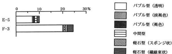
図1 火山ガラス比ダイアグラム
