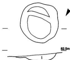
第11図 S002平面・断面図（1/30）
