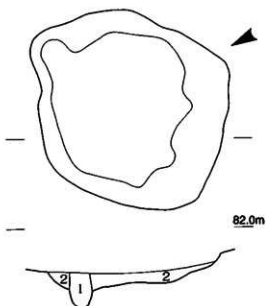
第14図 S005平面・断面図 (1/30)
