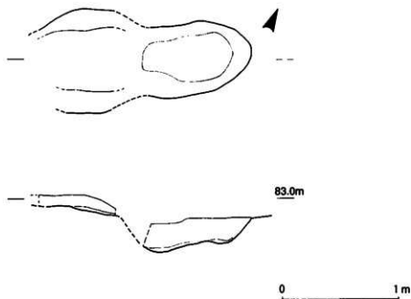
第9図 S100平面・見通し図 (1/30)
