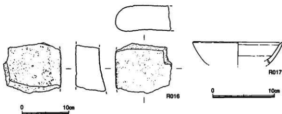
第21図 遺物実測図②
