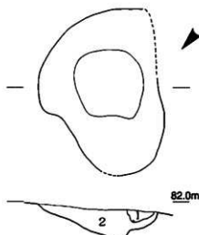
第12図 S003平面・断面図（1/30）
