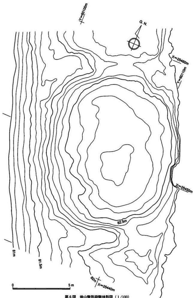
第6圖 地山盤形段階地形圖 (1/100)
