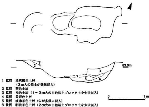
第10図 S101平面・断面図 (1/30)
