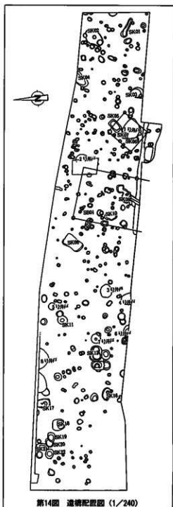
第14図 遺構配置図 (1/240)
