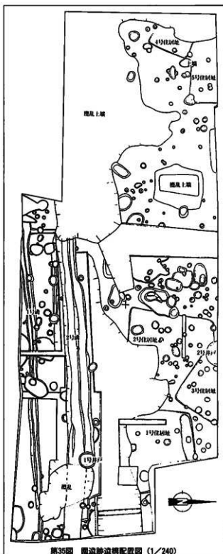
第35図 遺跡跡遺構配置図 (1/240)
