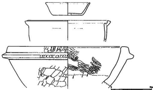
第15図 出土土器実測図 (1/4)
