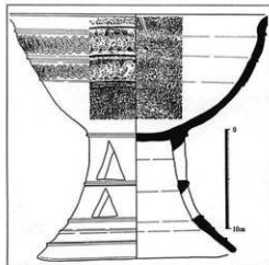
第7図 出土器台実測図 (1/4)
