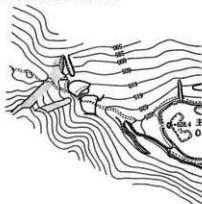
第45図 高崎山城跡遺構配置図
