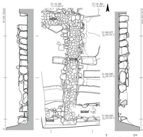
Fig. 34 SD330側石立面図 1:80
