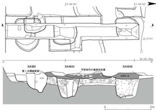
Fig. 29 SA4645・4646柱穴断面図 1:50
