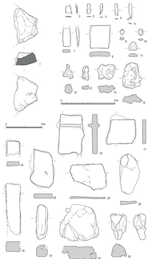
Fig. 133 石神遺跡第1～4次調査出土埴塼 1：3、銅素材・銅滴・銅滓・鉄素材 1：2
