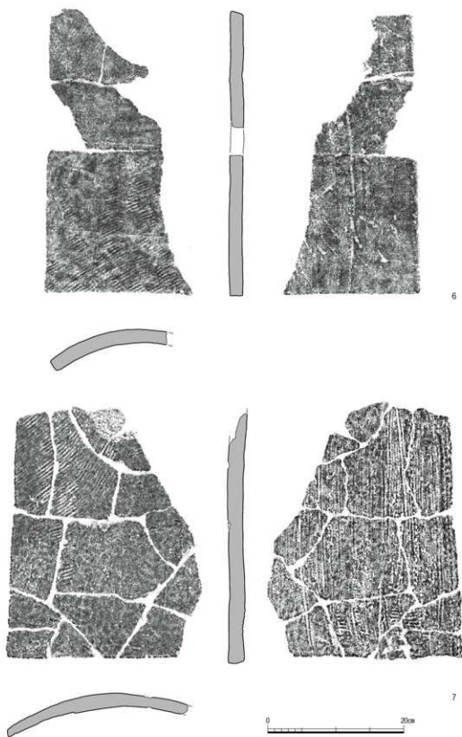
Fig. 85 平瓦 2 類 B 1:5
