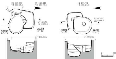
Fig. 37 SB736・750柱穴断面図 1:80
