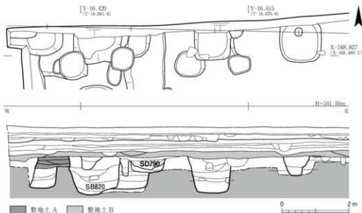
Fig. 26 SB810柱穴断面図 (第4次調査区北壁土層図) 1:80
