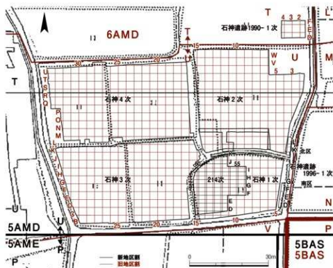
Fig. 8 第1～4次調査区周辺の地区割 1:1,000
