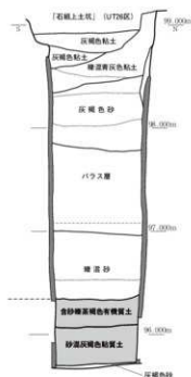
Fig. 44 SE800井戸枠内の層位 1:40
