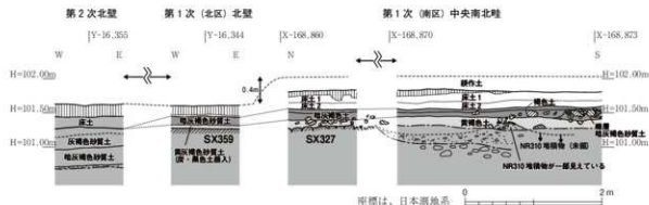
Fig.17 第1・2次調査区の層序(柱状図) 1:60
