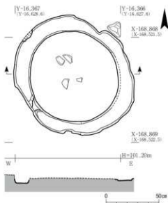
Fig. 43 SX350平面図・断面図 1:25
