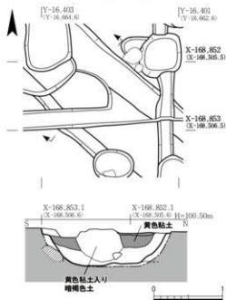
Fig. 42 SD577平面図・断面図 1:50
