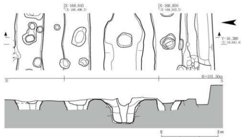
Fig. 31 SB735の布掘り工法 1:100
