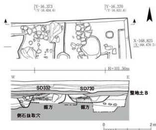
Fig. 38 SD332・730断面図 1:80
