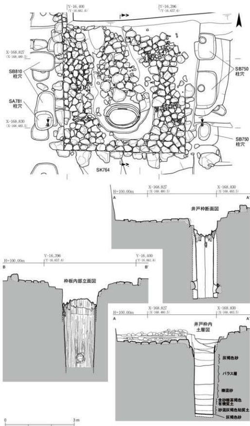
Fig. 27 SE800平面図および東西・南北断面図 1:80
