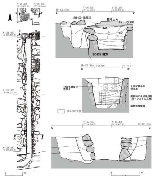
Fig. 23 SD335断面図 1:40 (断面位置図は1:200)
