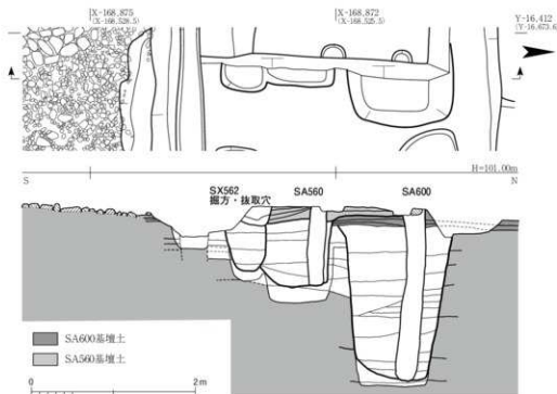
Fig. 21 SA600・560基壇土断面図 1:50
