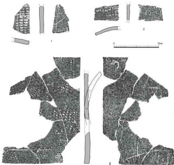
Fig. 83 平瓦1類 1:5
