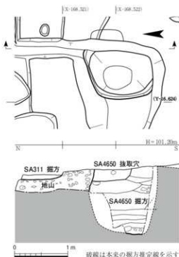
Fig. 22 SA4650柱穴断面図 1:50
