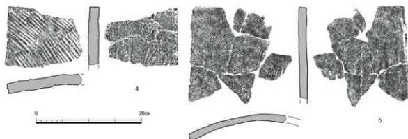
Fig. 84 平瓦2類A 1:5
