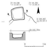
Fig.40 SA311柱穴断面図 1:50
