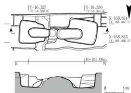
Fig. 28 SA1460柱穴断面図 1:100
