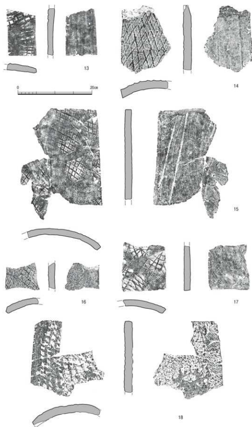
Fig.88 平瓦 4類 1:5
