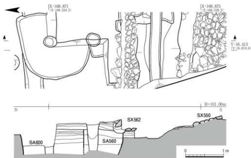
Fig. 36 石敷SX550とSA560基壇外装SX562断面図 1:50
