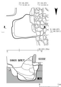
Fig.33 SB620柱穴断面図 1:50
