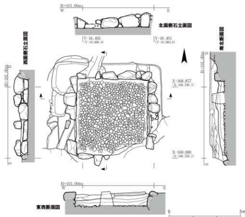
Fig. 39 SX540断面図および立面図 1:80
