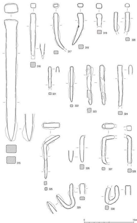
Fig.121 第1～4次調査出土鉄釘(1) 1:2
