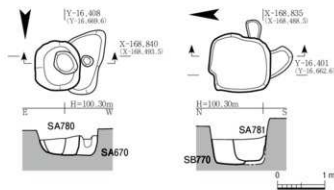
Fig. 41 SA780・781柱穴断面図 1:80
