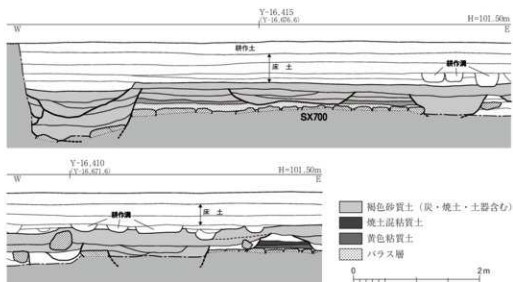
Fig. 18 第3次調査区北壁土層図(部分) 1:60
