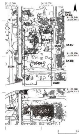
Fig. 32 SB400と周辺の石敷・石列 1:300
