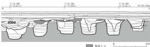
Fig. 25 SB750柱穴断面図 1:100
