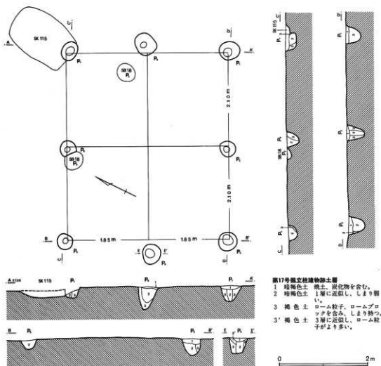
第138図 第17号掘立柱建物跡
