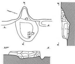
第91図 第31号住居跡カマド
