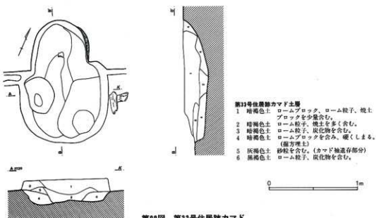
第99図 第33号住居跡カマド
