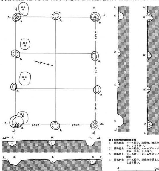
第121図 第4号掘立柱建物跡
