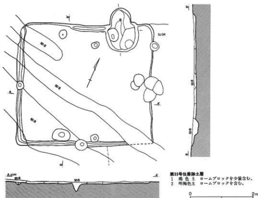
第98図 第33号住居跡
