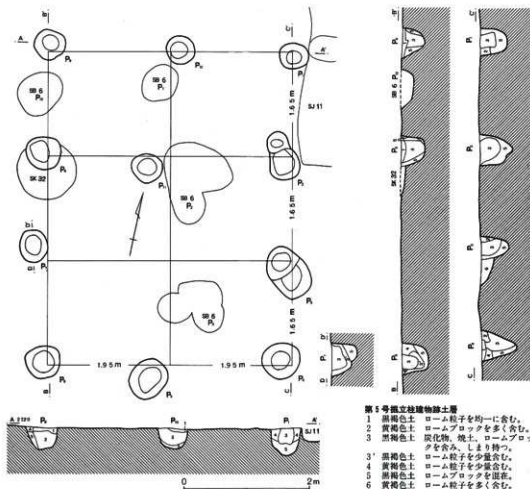
第123図 第5号掘立柱建物跡
