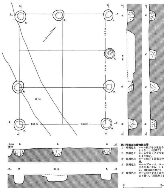
第154図 第31号掘立柱建物跡
