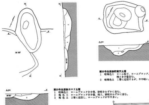
第105図 第35号住居跡カマド・貯蔵穴
