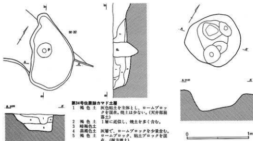
第102図 第34号住居跡カマド・貯蔵穴
