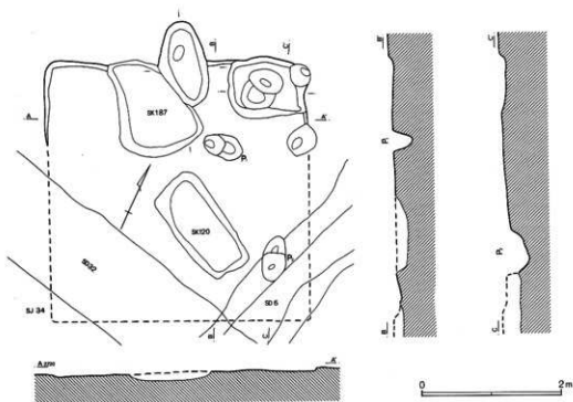
第104図 第35号住居跡
