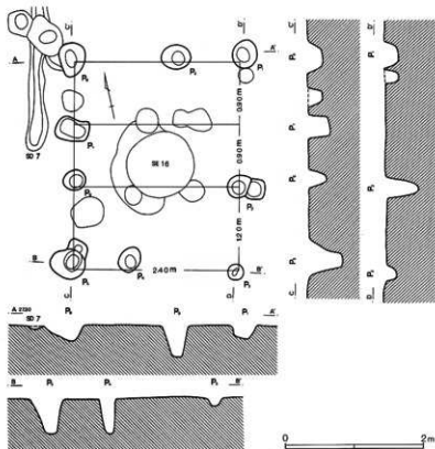
第132図 第11号掘立柱建物跡
