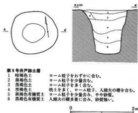
第165図 第9号井戸跡
