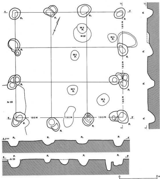
第125図 第6号掘立柱建物跡
