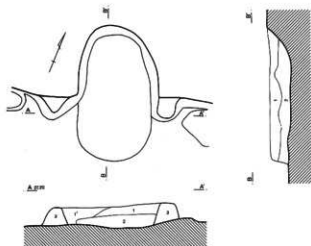
第107図 第36号住居跡・カマド
