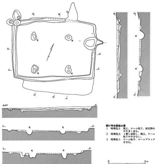
第90図 第31号住居跡
