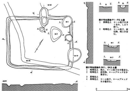
第109図 第37号住居跡・住居内1、2号土層
