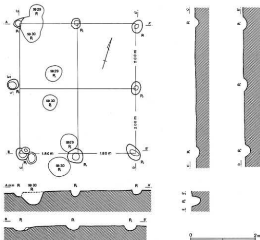
第151図 第28号掘立柱建物跡
