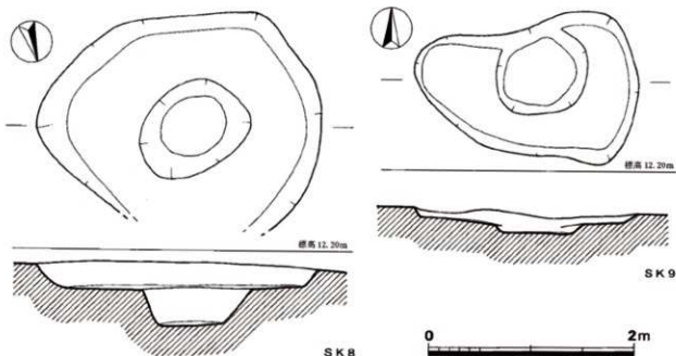
第10図 SK8・9実測図（1/40）
