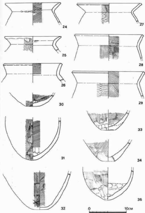
第28図 S D 4 出土遺物実測図③ (1/5)
