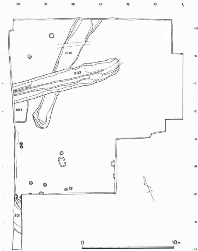
第21図 第3次調査遺構配置図 (1/50)
