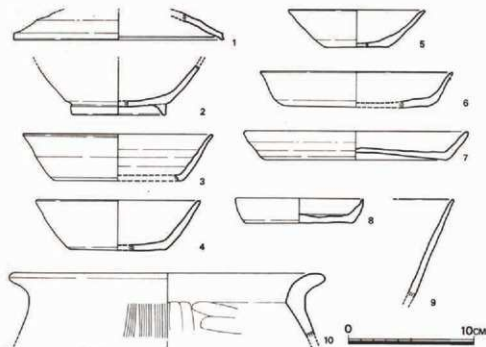
第18図 G-02区出土遺物実測図(1/5)
