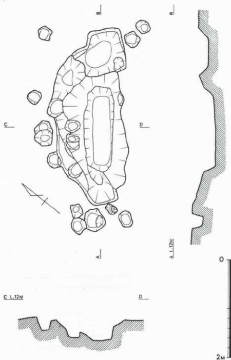
第34図 SK10・11道橋実測図 (1/6)
