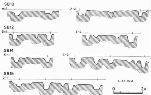
第36図 掘立柱建物址断面図 (1/40)
