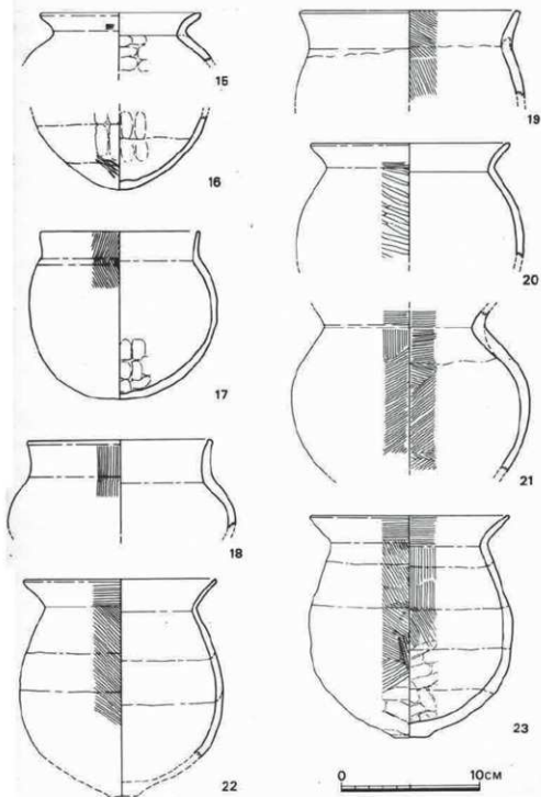
第27図 SD 4 出土遺物実測図② (1/4)
