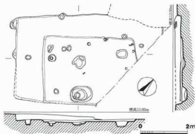
Fig.5 SI160実測図 (1/80)
