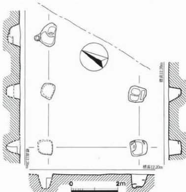
Fig.10 S B 100実測図 (1/80)
