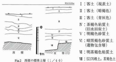
Fig.2 西壁の標準土層 (1/40)
