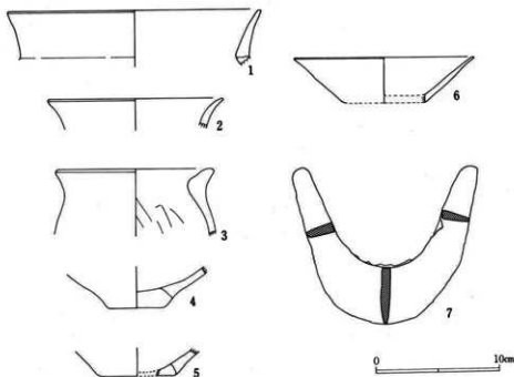
第7図 D地点出土遺物
