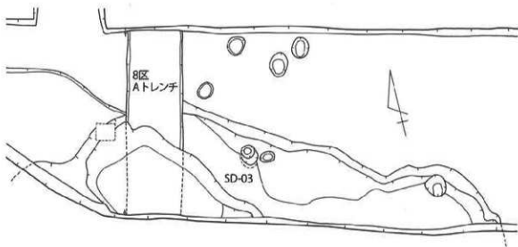
第28図 第8区 SD-03 実測図 (S=1/60)
