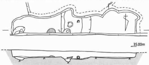
第75図 SB-09 実測図 [S=1/40]
