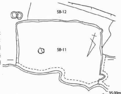
第77図 SB-11 実測図 [S=1/40]
