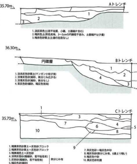
第26図 第7区 A～Cトレンチ 土層断面図 [S=1/40]
