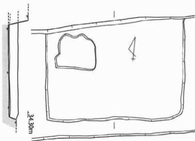
第20図 SB-01 実測図 [S=1/60]
