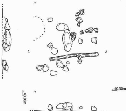
第106図 SB-01 石組部 実測図 [S=1/40]
