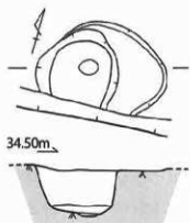
第73図 SK-05 実測図 [S=1/40]
