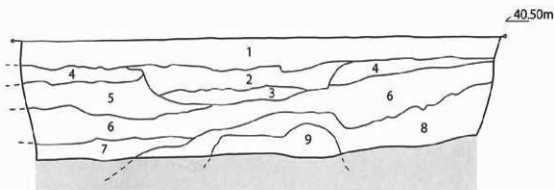
第103図 SD-01 No.1トレンチ 西側土層 実測図 (S=1/40)
