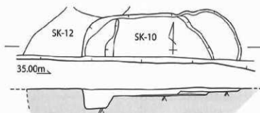
第81図 SK-10 実測図 (S=1/40)
