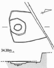
第21図 SK-01 実測図
