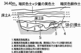
第60図 早水町遺跡 A区 SK-02 西側土層断面図 [S=1/40]
