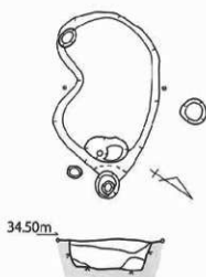
第12図 SK-02実測図 [1/40] 2地点
