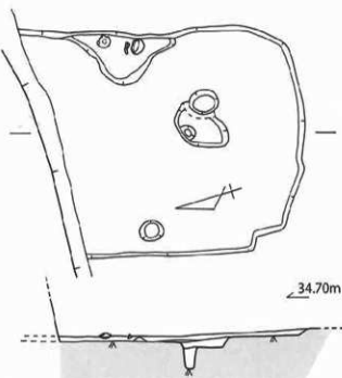
第70図 SB-07 実測図 [S=1/40]
