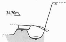
第72図 SK-02・03 実測図 [S=1/40]
