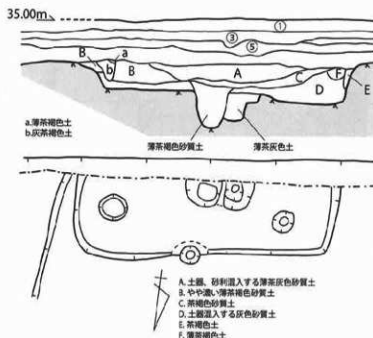
第7図 SB-02実測図〔1/40〕
