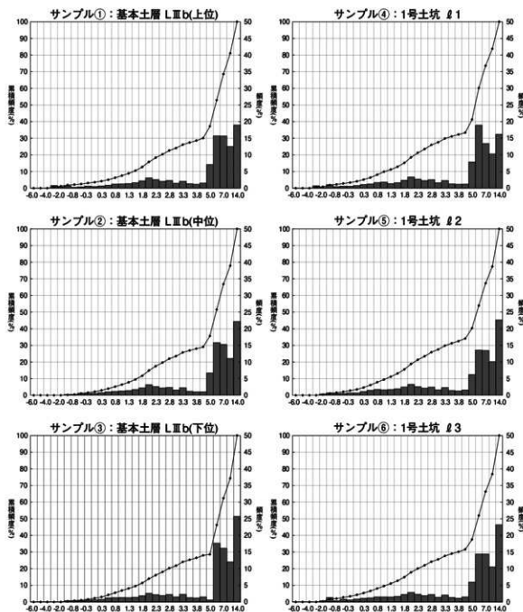
図 25 粒度組成
