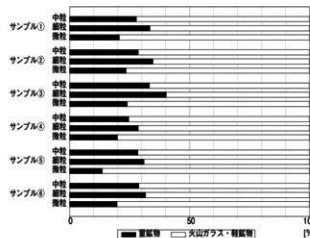
圖 26 重輕鮫物比
