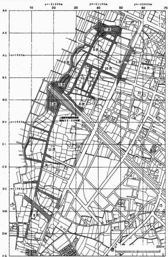
第3図 遺跡周辺の地形図
