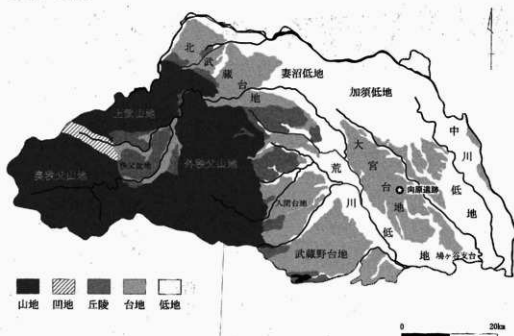
第1図 埼玉県の地形図
