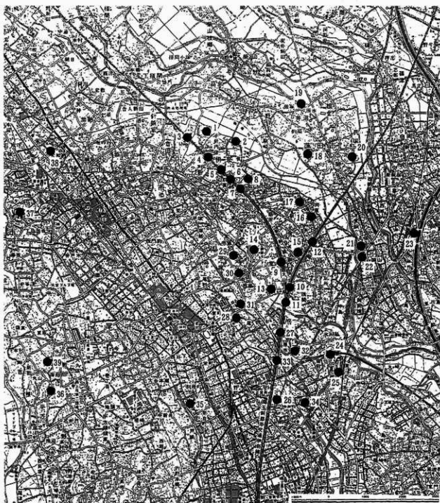
第2図 周辺の遺跡分布図
