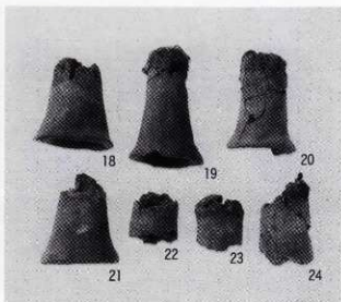
羽口 (4)
