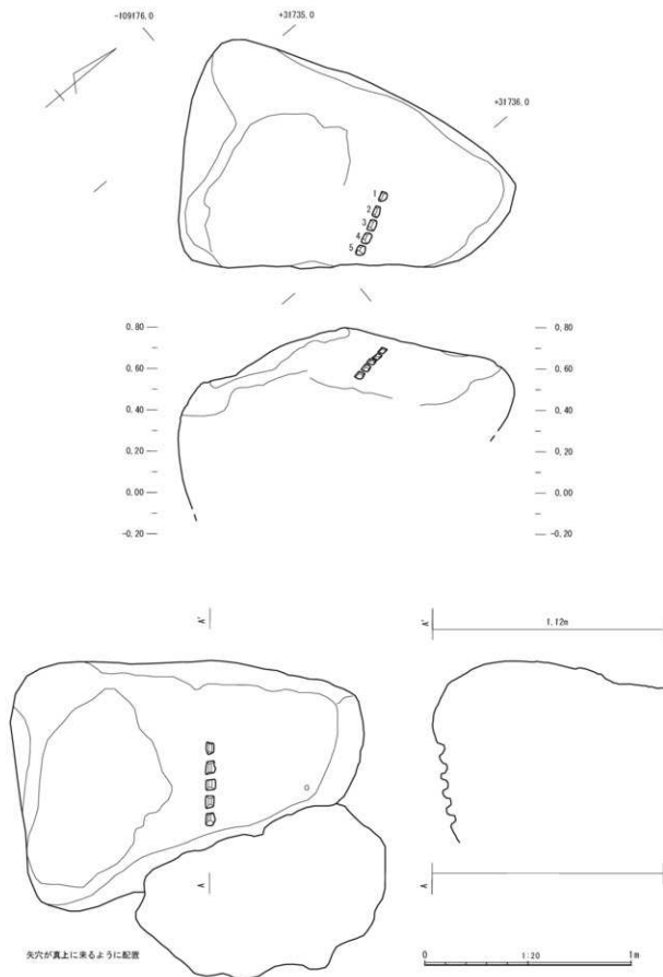
第7図 矢穴石3平面図・立面図
