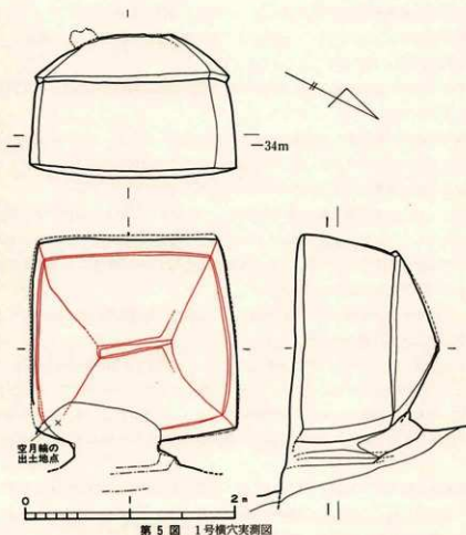
第5図 1号横穴実測図
