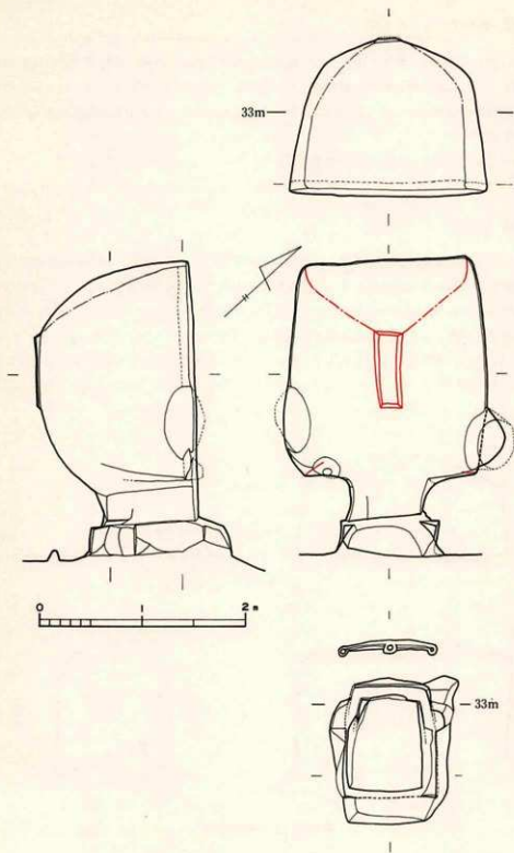
第 11 图 9 号横穴夷测图
