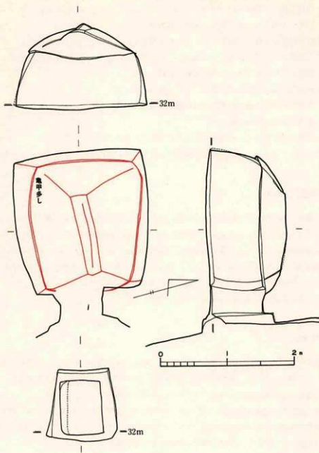
第 19 図 18号横穴実測図
