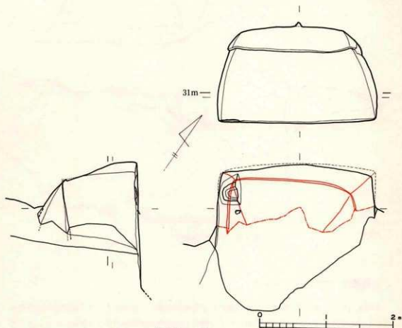
第7図 4号横穴実測図
