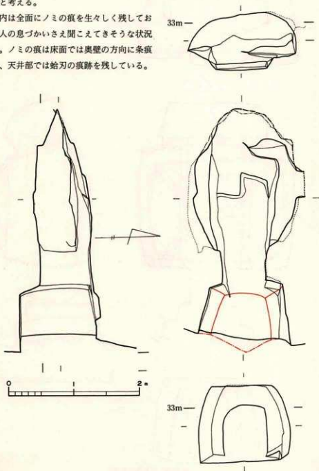
第20図 19号横穴実測図
