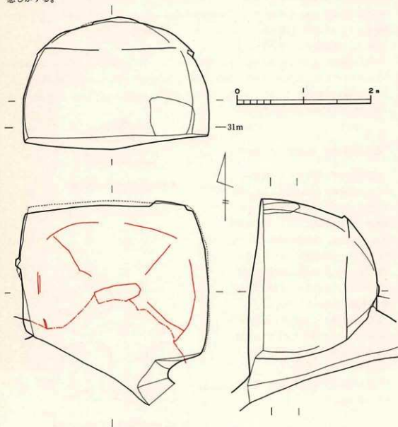
第48図 43号横穴実測図
