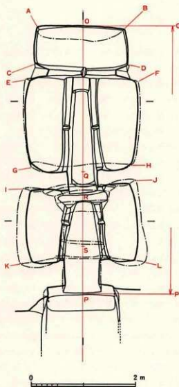
第 52 図 板の上 I - 2 号横穴実測図 (「熊本県装飾古墳総合調査報告書」より引用)
