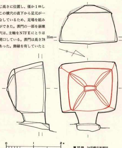
第37図 34号横穴実測図
