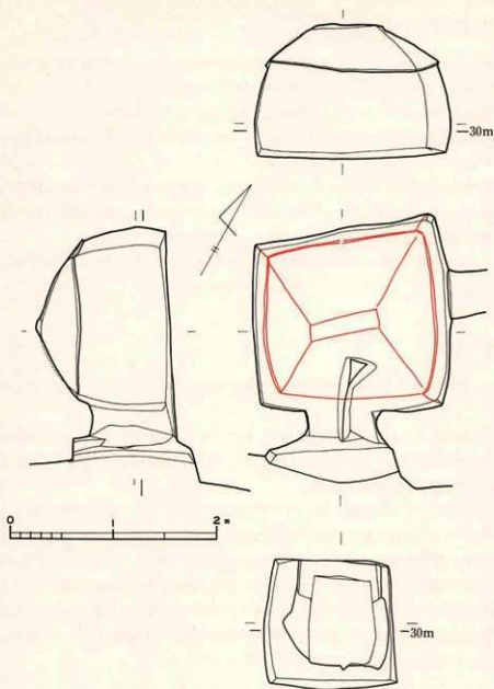
第12図 10号横穴実測図
