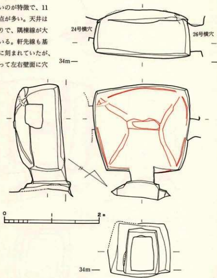
第27図 25号横穴実測図
