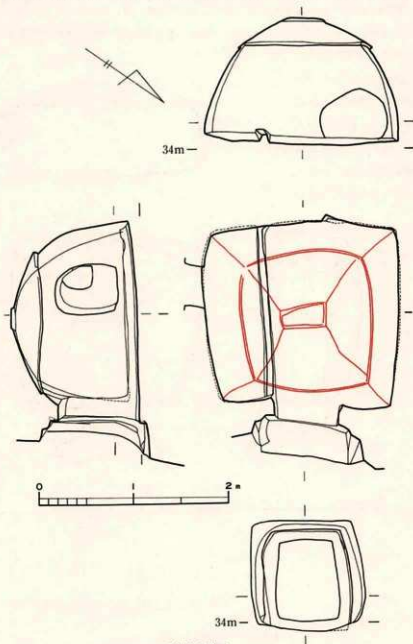
第28図 26号横穴実測図
