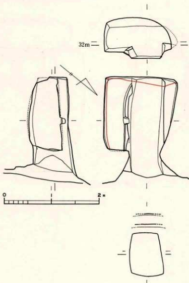
第15図 14号横穴実測図
