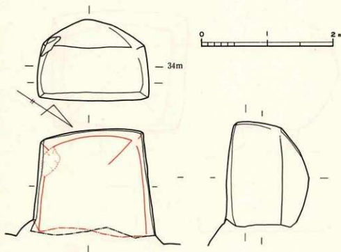
第31図 29号横穴実測図
