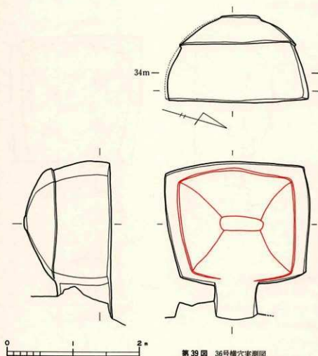
第 39 図 36号横穴実測図
