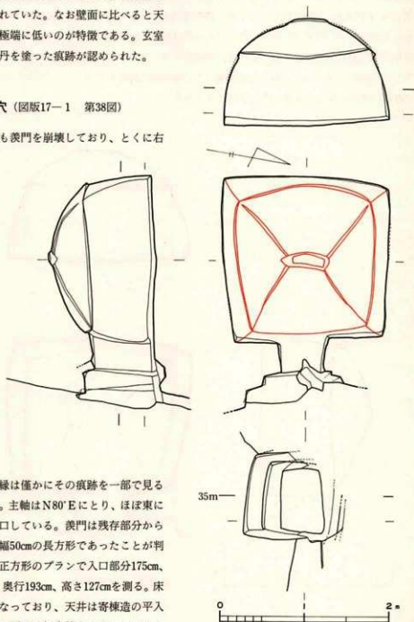
第38図 35号横穴実測図
