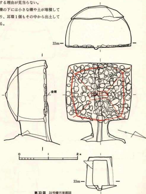
第33図 31号横穴実測図
