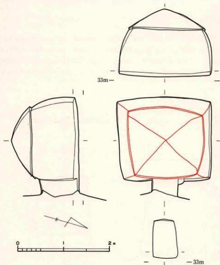
第32図 30号横穴実測図
