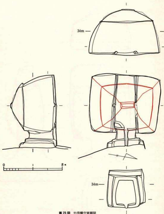
第 23 図 21号横穴実測図
