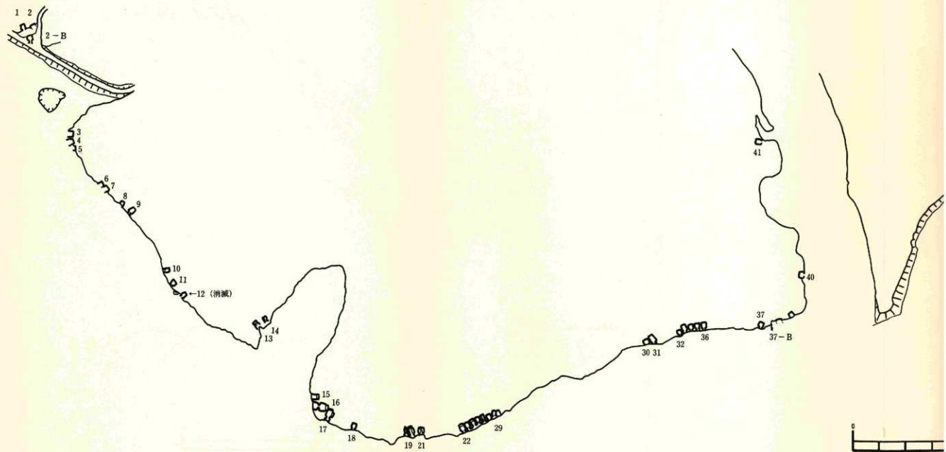
第 3 図 横穴配置図 (熊本県佐野古墳総合調査報告書より引用)
