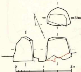
第47図 42-B号横穴実測図
