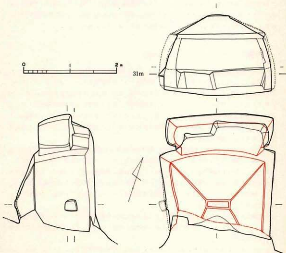
第16図 15号横穴実測図
