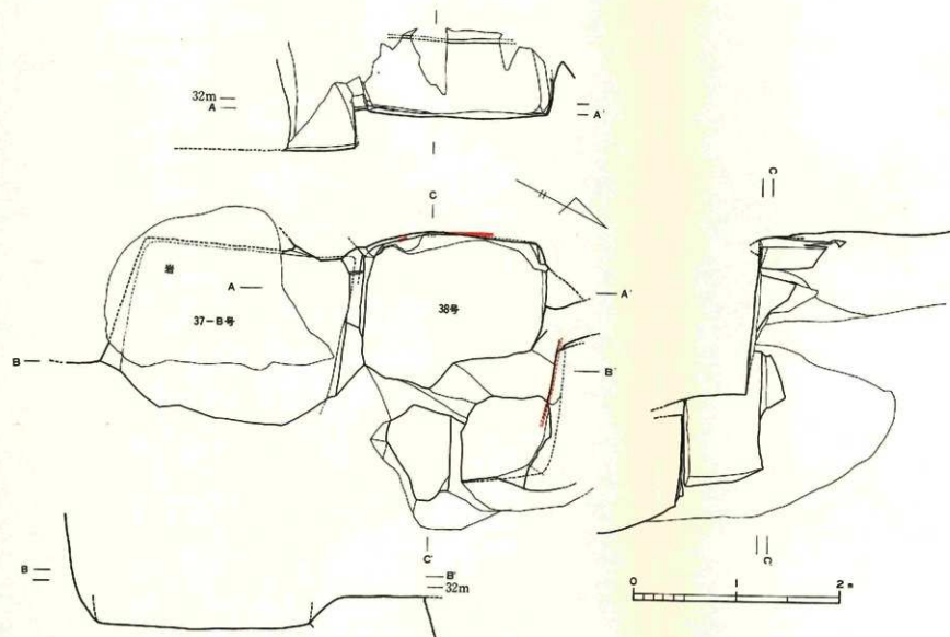
第41圖 37-B号横穴・38号横穴実測図
