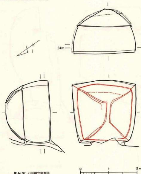
第44図 41号横穴実測図
