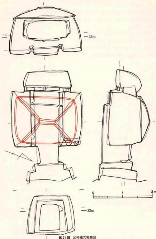
第 21 图 20号横穴夷洞图
