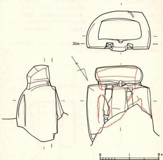
第 14 图 13号横穴实测图
