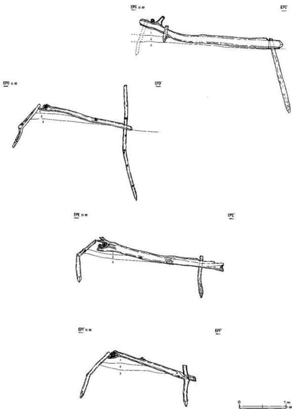
第307图 堰構梁材横断面图(1)
